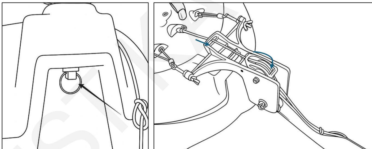
2-2. Installation du gouvernail
