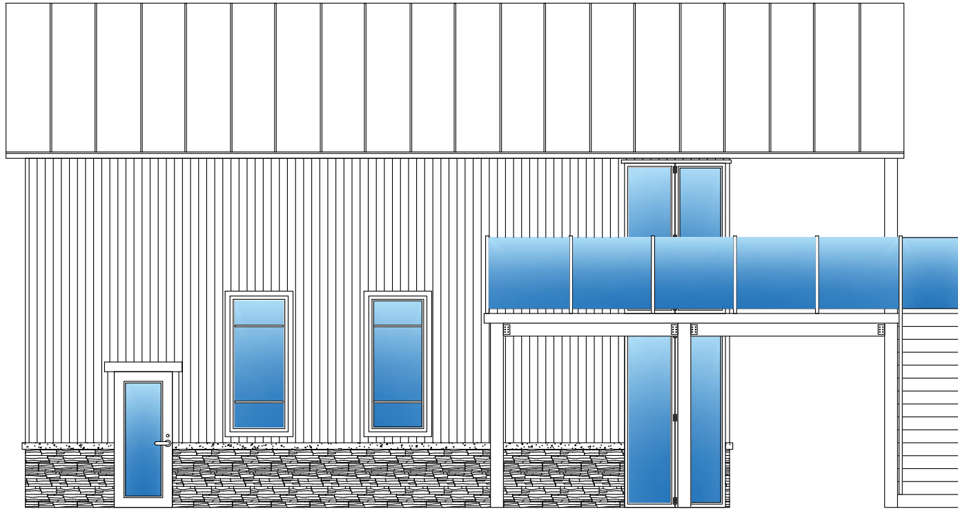
RIGHT ELEVATION
