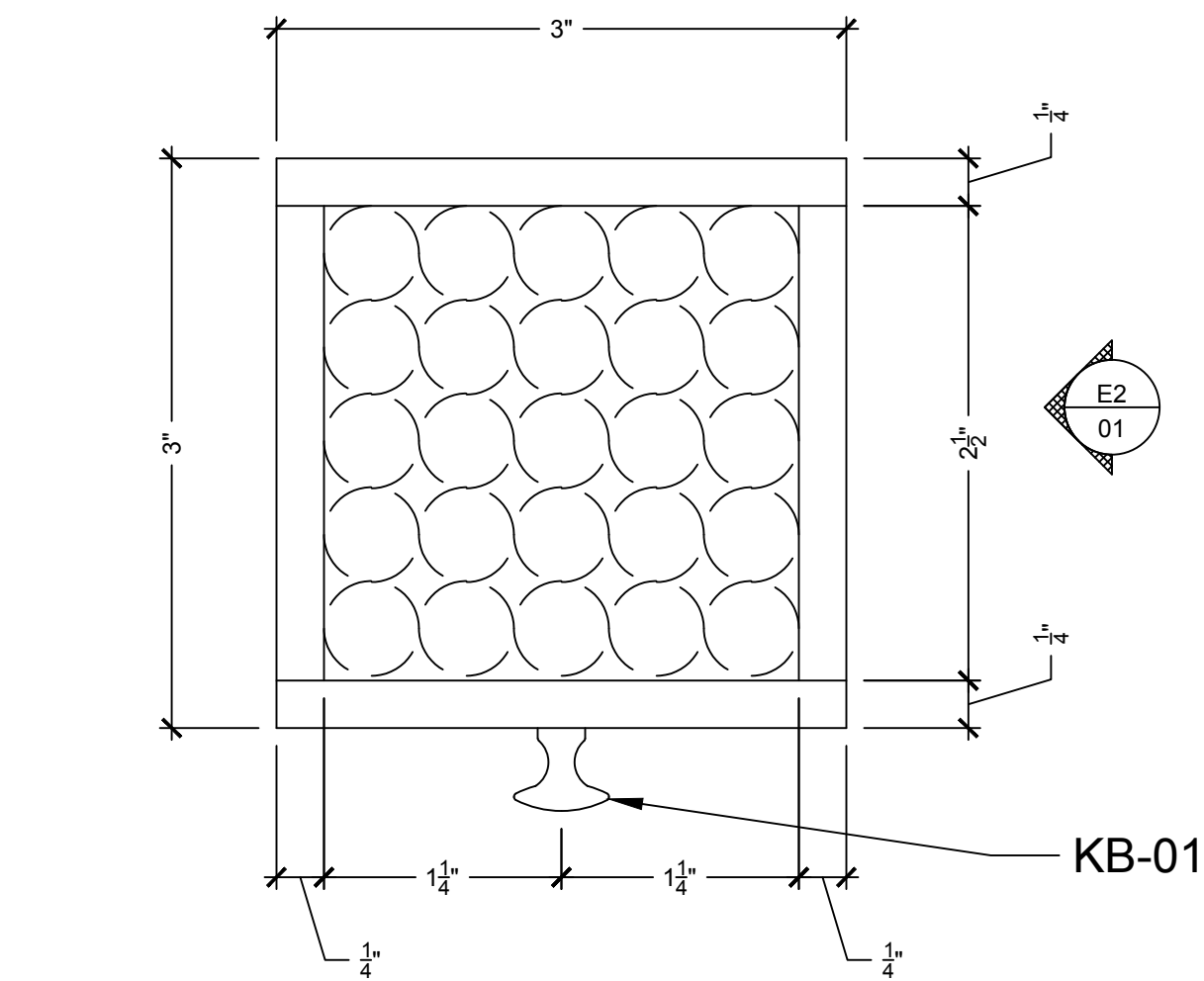
P1 01 PLAN: SHAKER CANDLE BOX SCALE: 12" = 1'-0"
