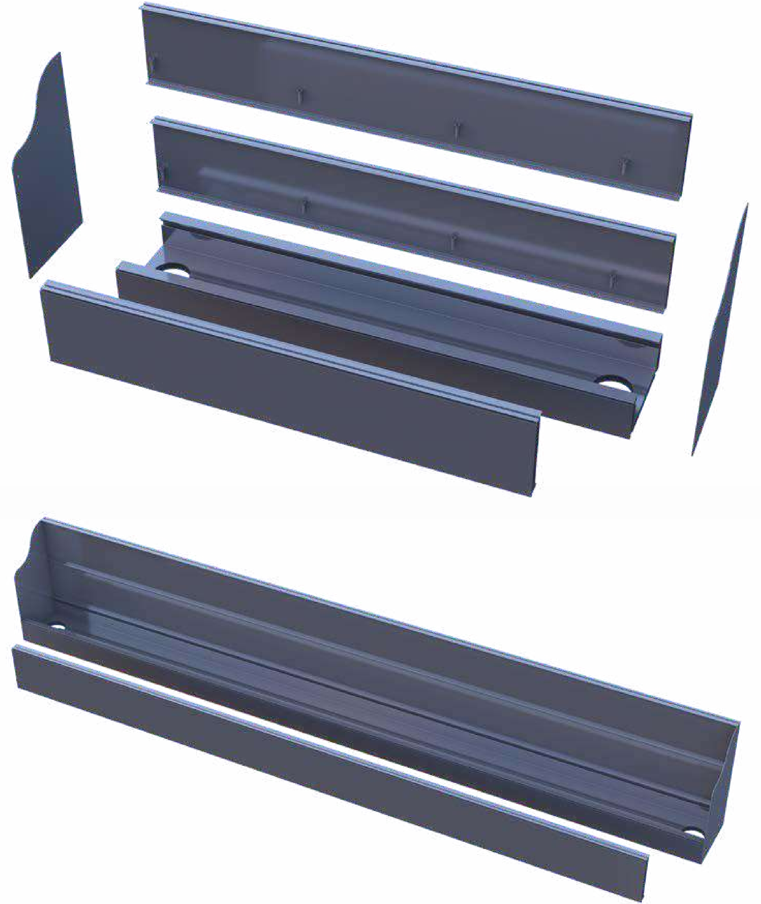
OLUK MONTAJ ŞEMASI / GUTTER INSTALLATION SCHEME
