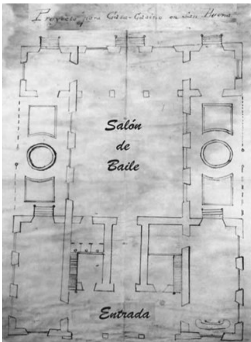
Plano original de lo que fue el proyecto de la Casa-Casino de San Buenaventura, Coah. -Circa 1906.45
