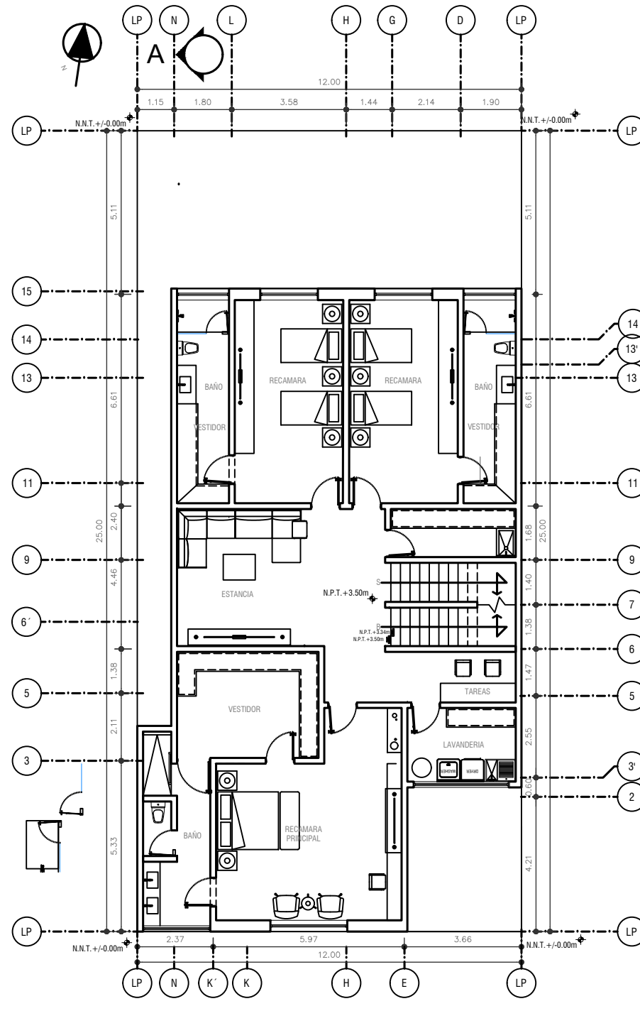
1N PLANTA ARQUITECTONICA PRIMER NIVEL
