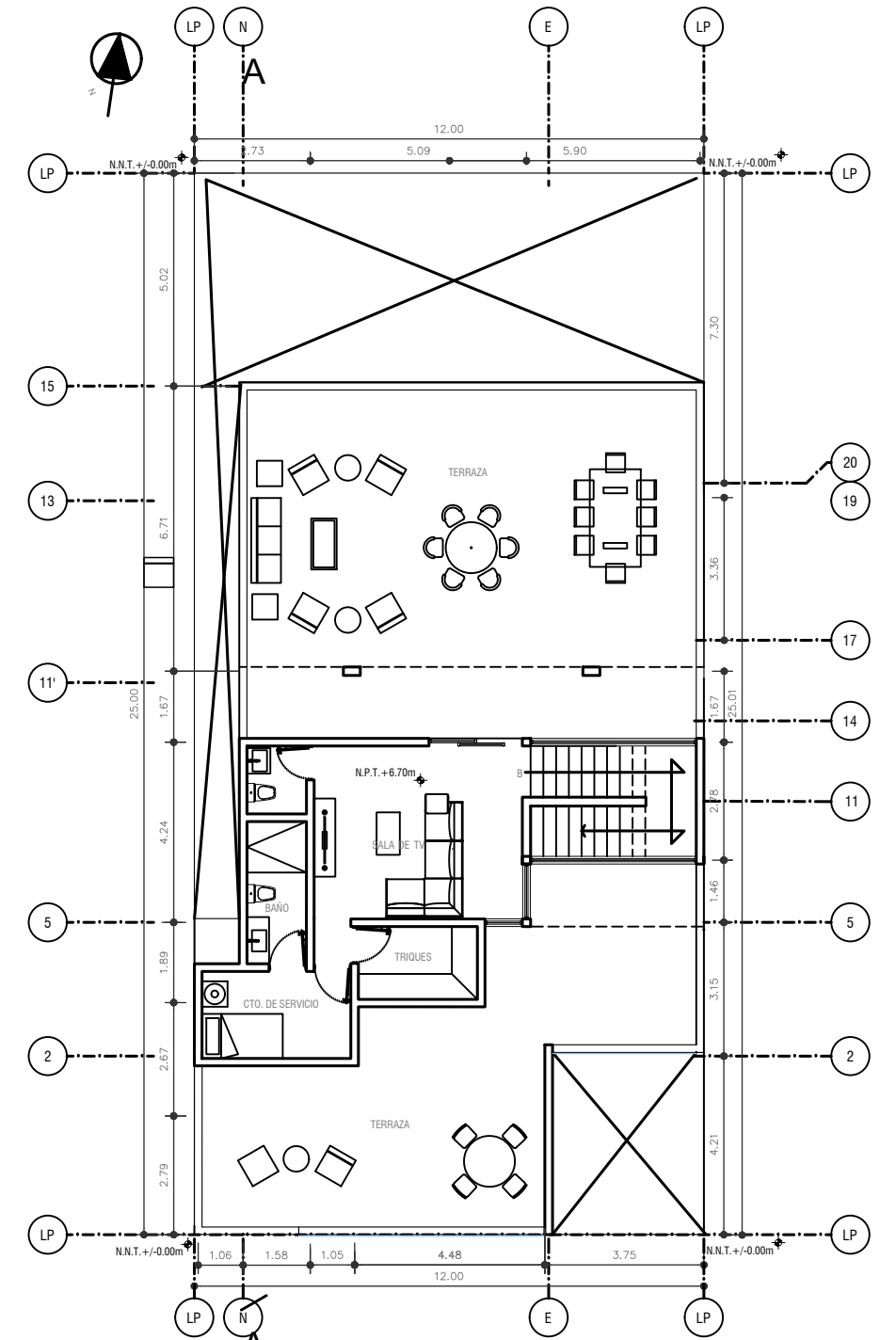
2N PLANTA ARQUITECTONICA SEGUNDO NIVEL
