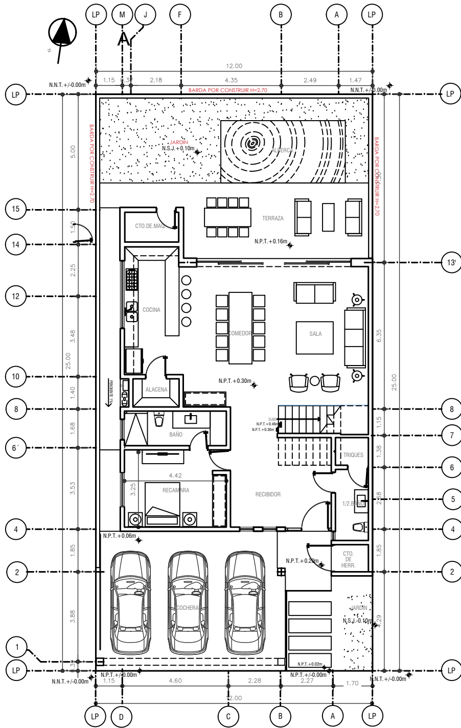
PB PLANTA ARQUITECTONICA PLANTA BAJA
