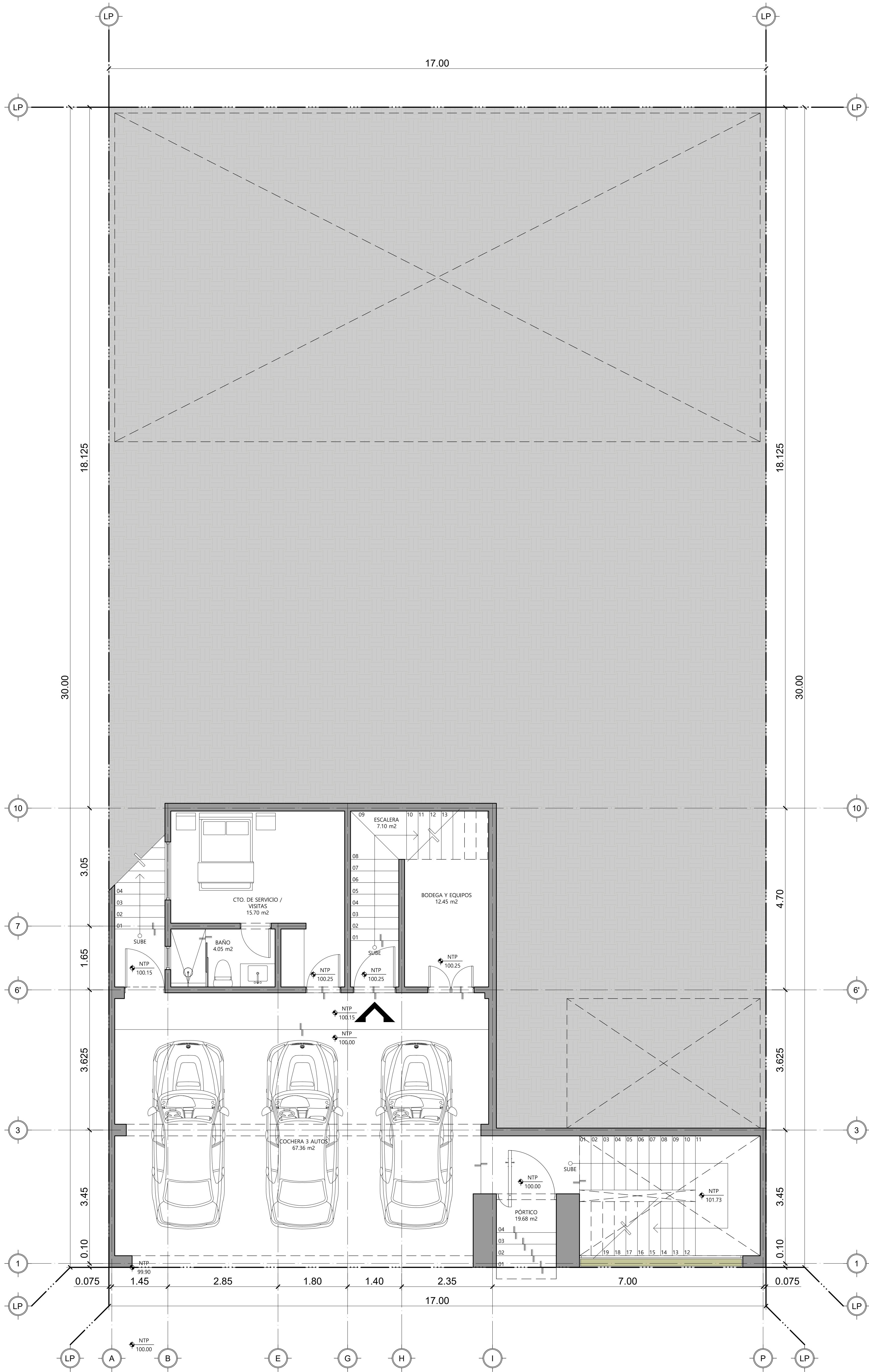
PLANTA BAJA 132.60 m 2 Total=637.14 m 2
