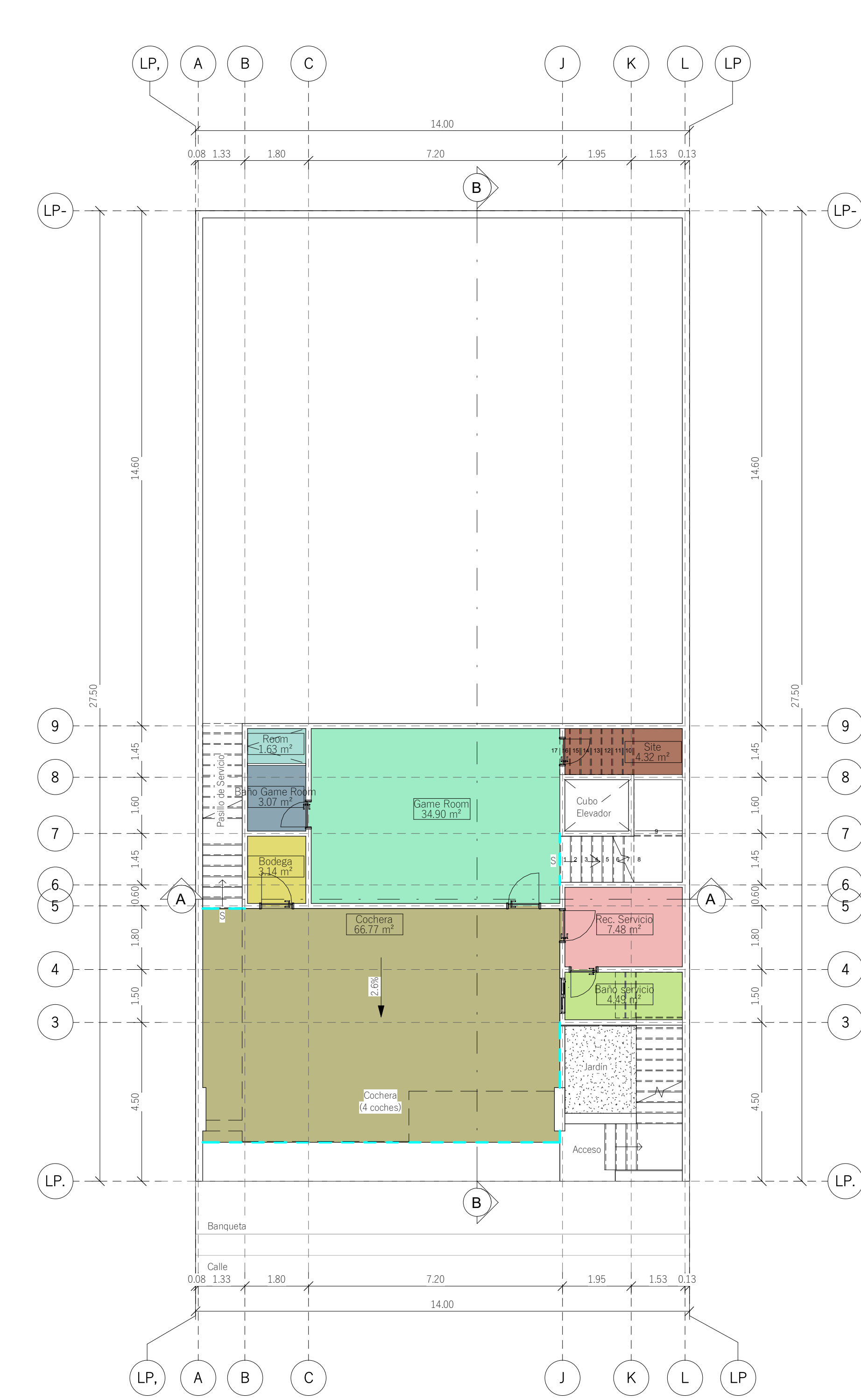
1 Sotano - área A104 | 1 : 100
