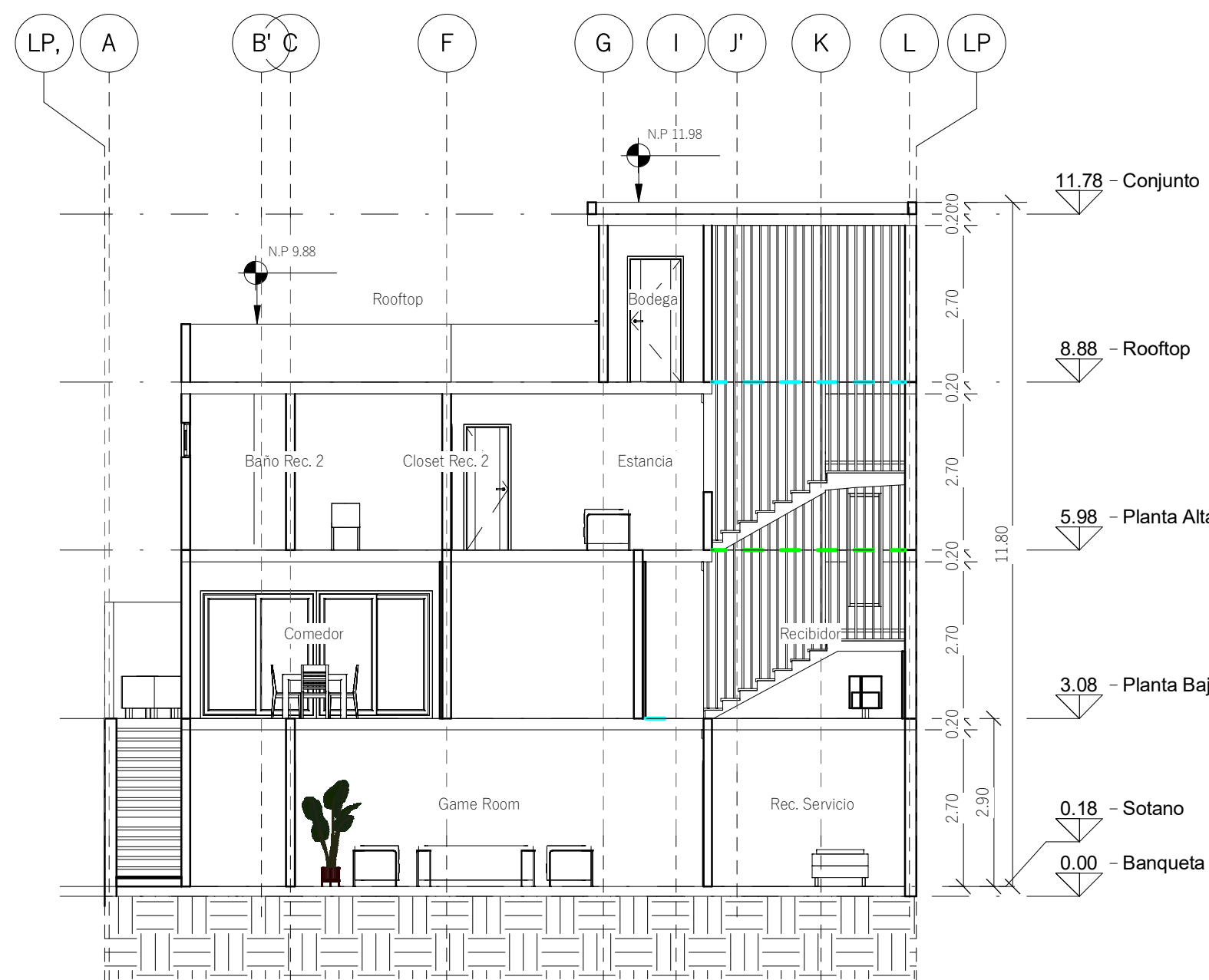
A Sección 1 A103 1:100
