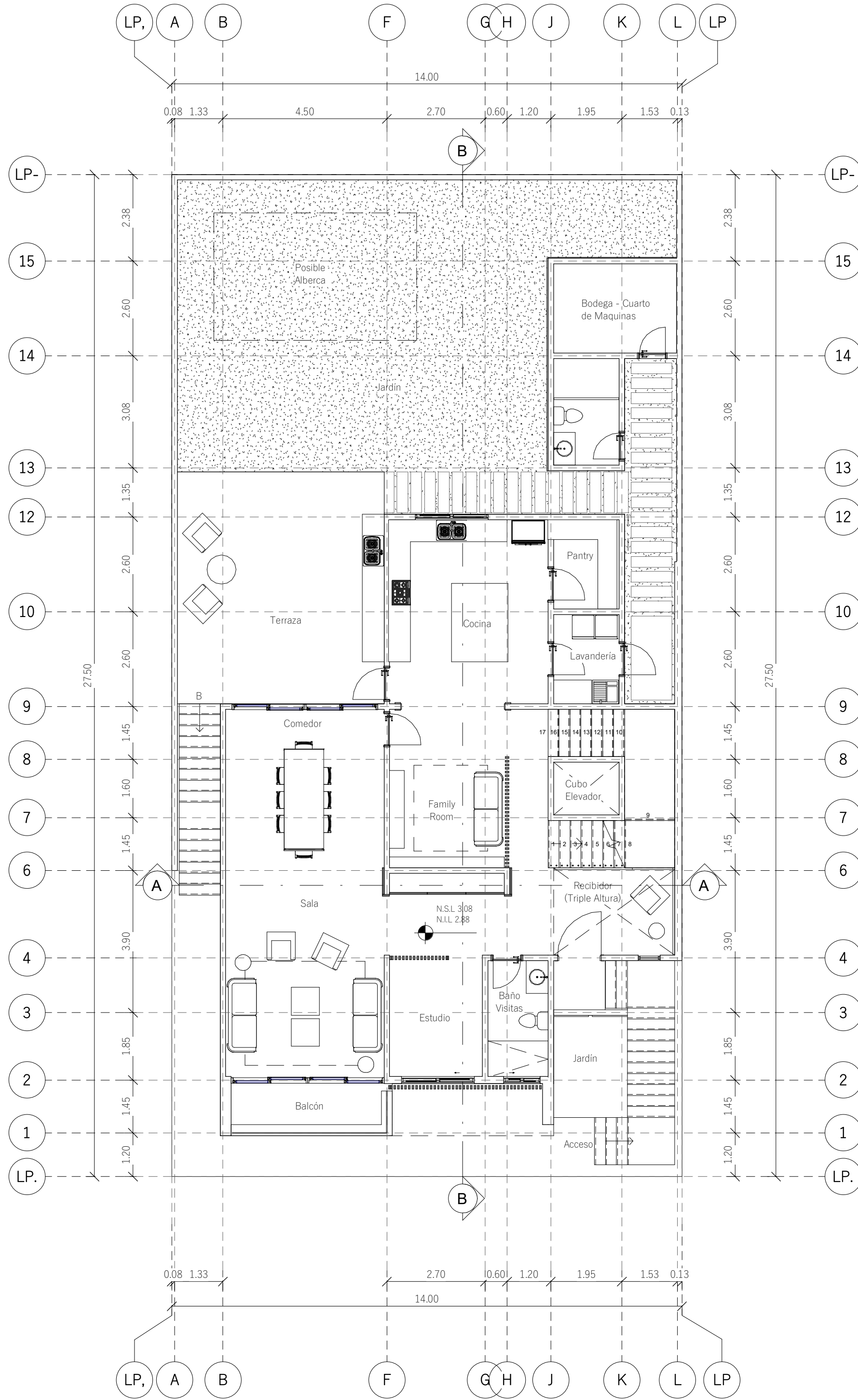
2 Planta Baja A101 1:100 198.63m2
