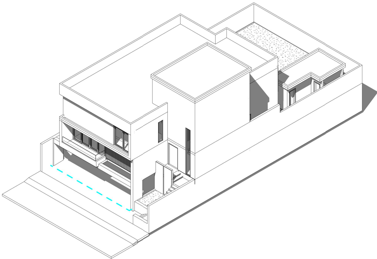
4 Isometría Sur A102
