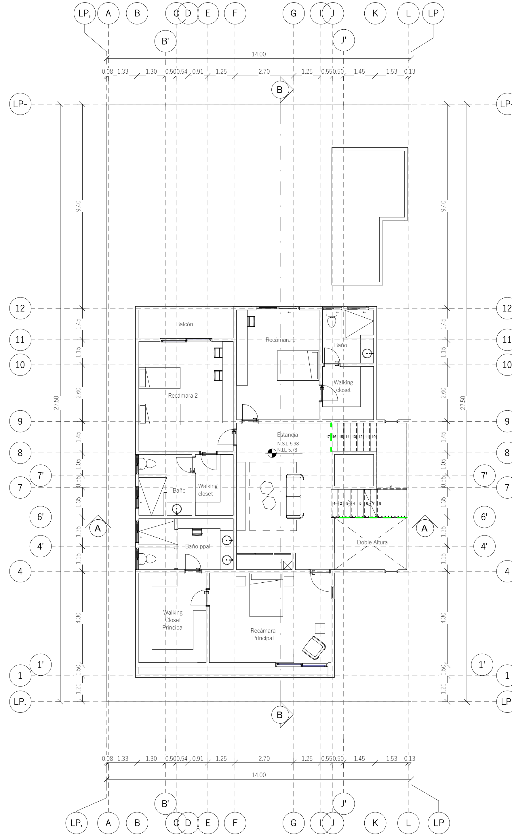
3 Planta Alta A101 1:100 174.00m2
