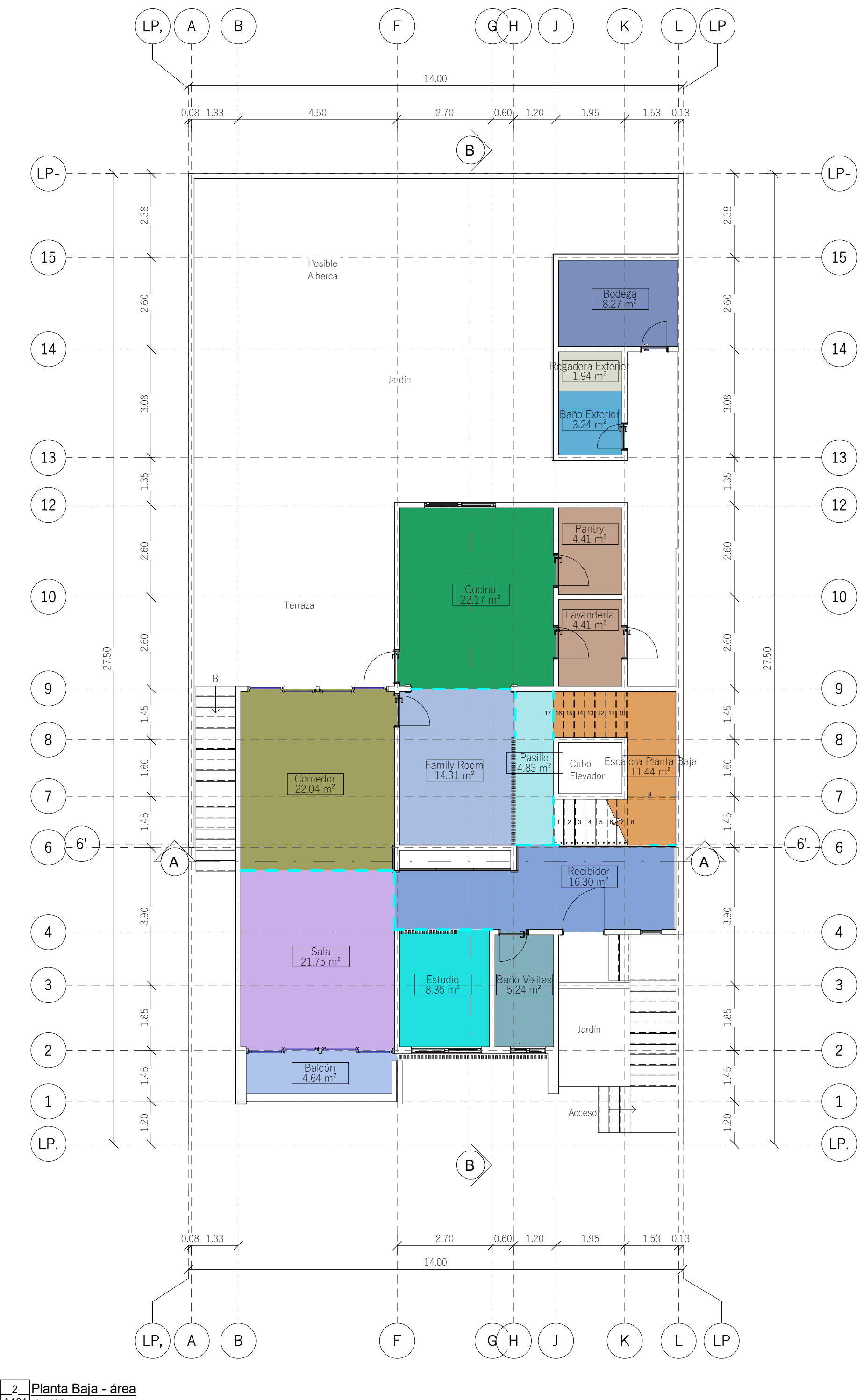
2 Planta Baja - área A104 | 1 : 100
