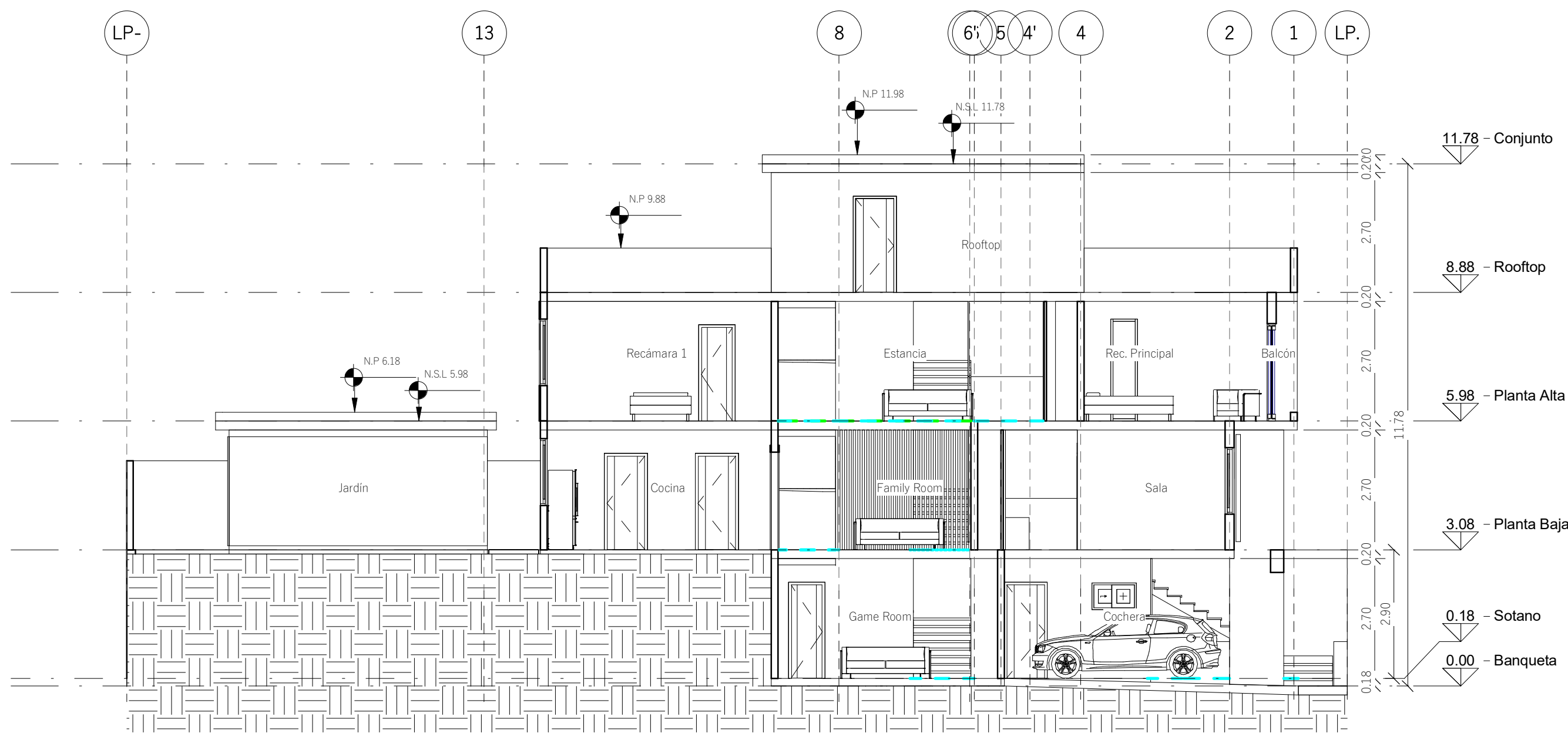
B Sección 2 A103 1:100
