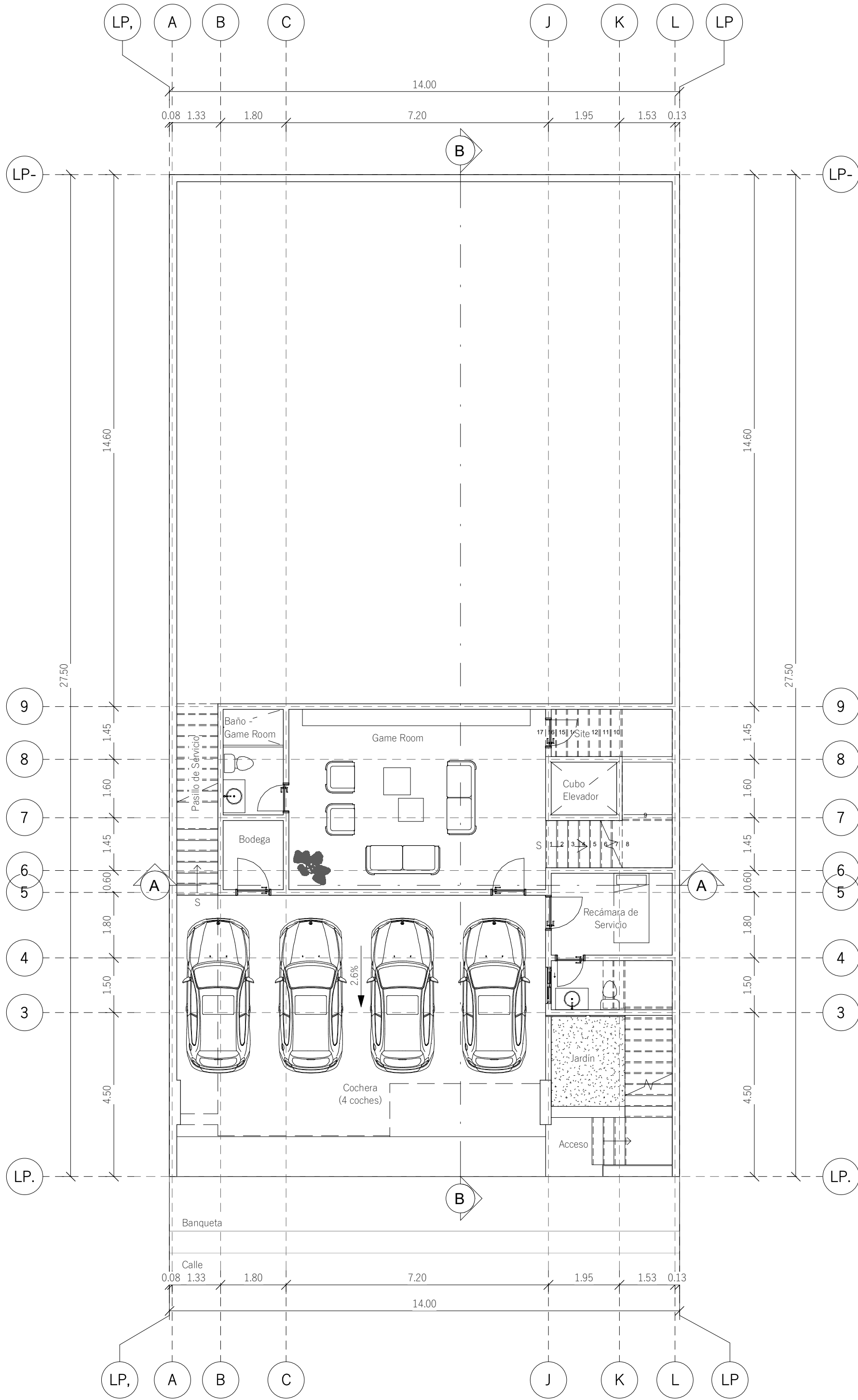
1 Sotano A101 1:100 128.60m2
