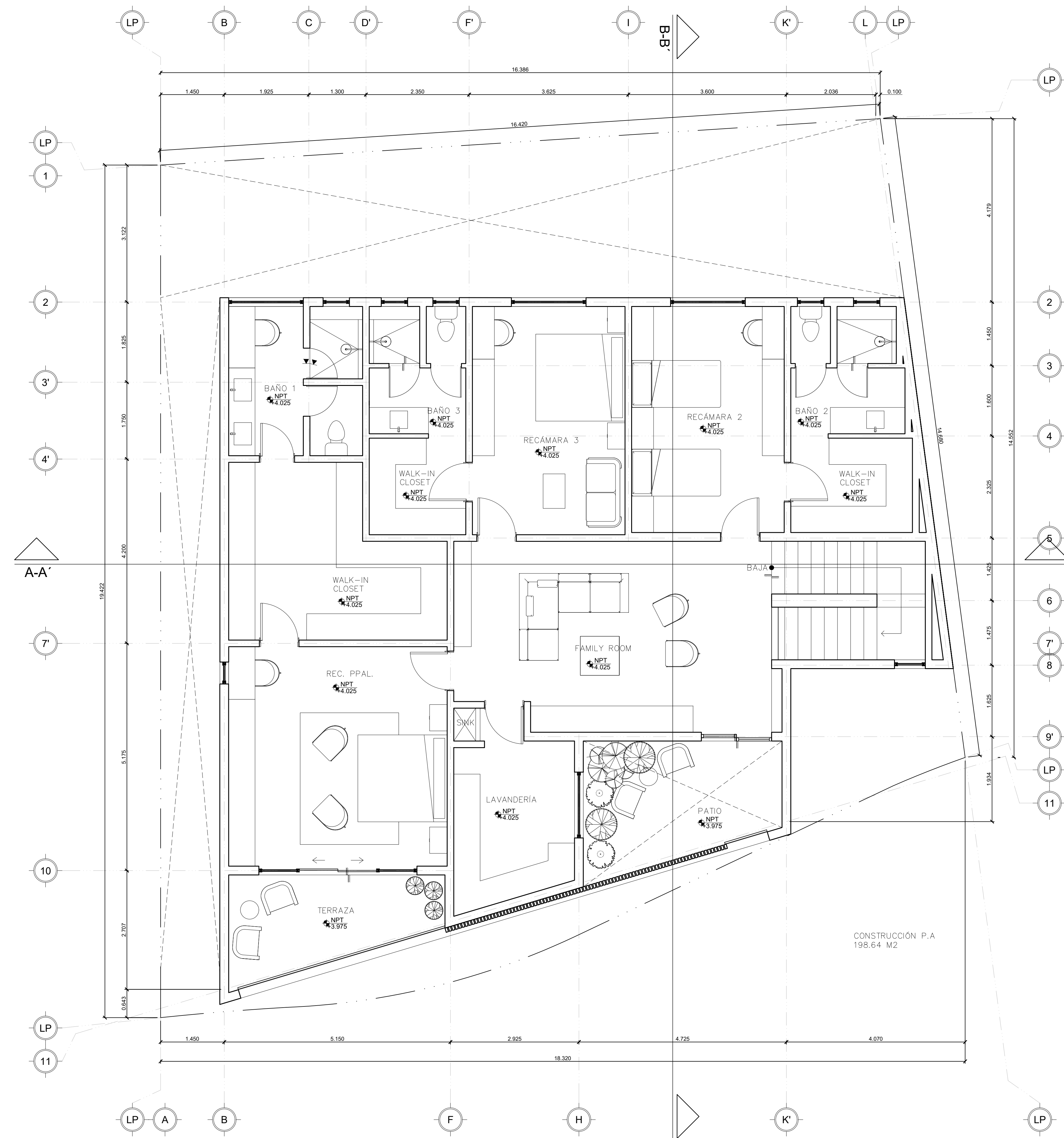
PLANTA ALTA ALMENA II
