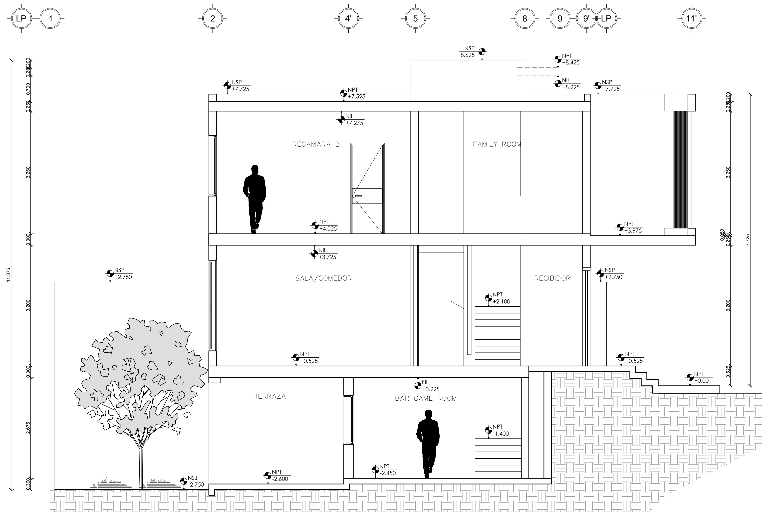
SECCION B-B'
