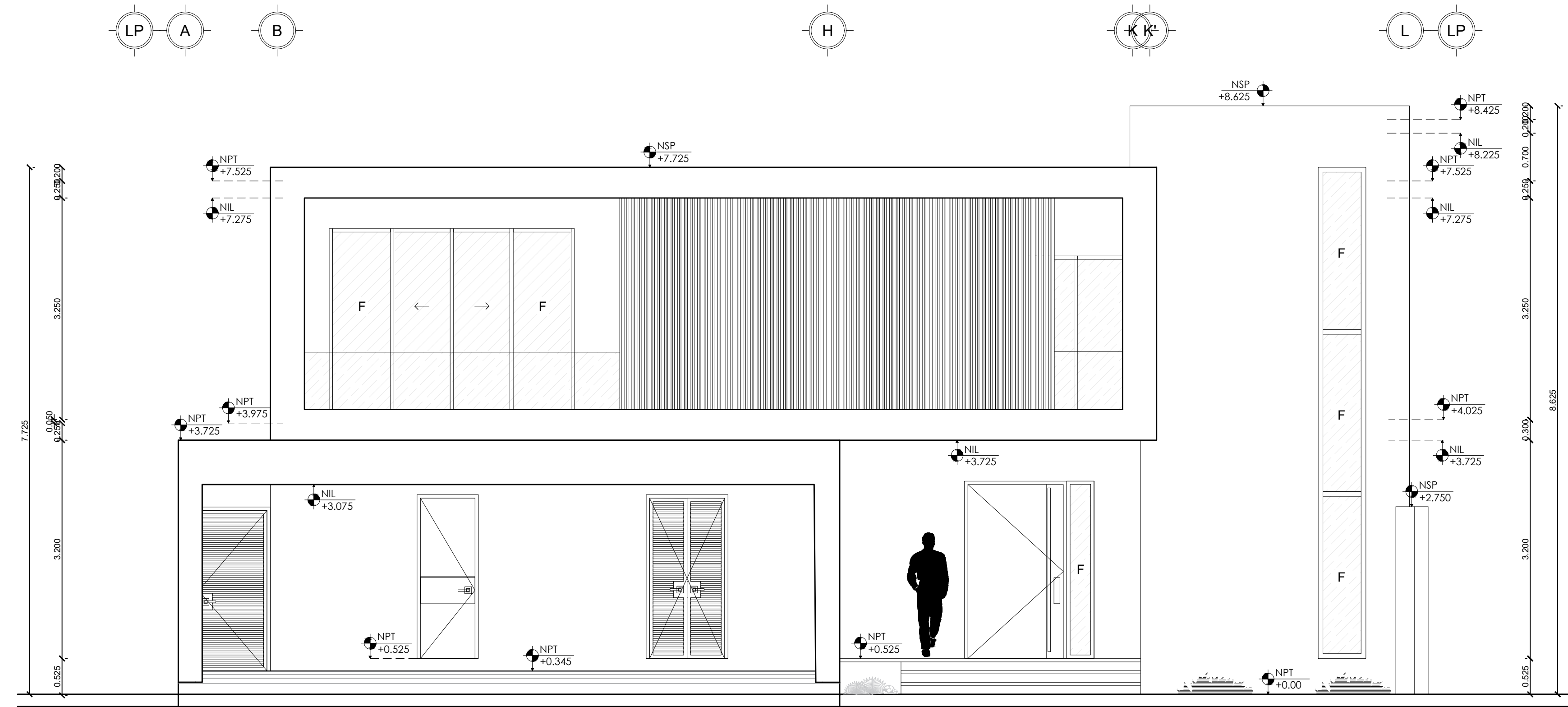
ELEVACION PRINCIPAL
