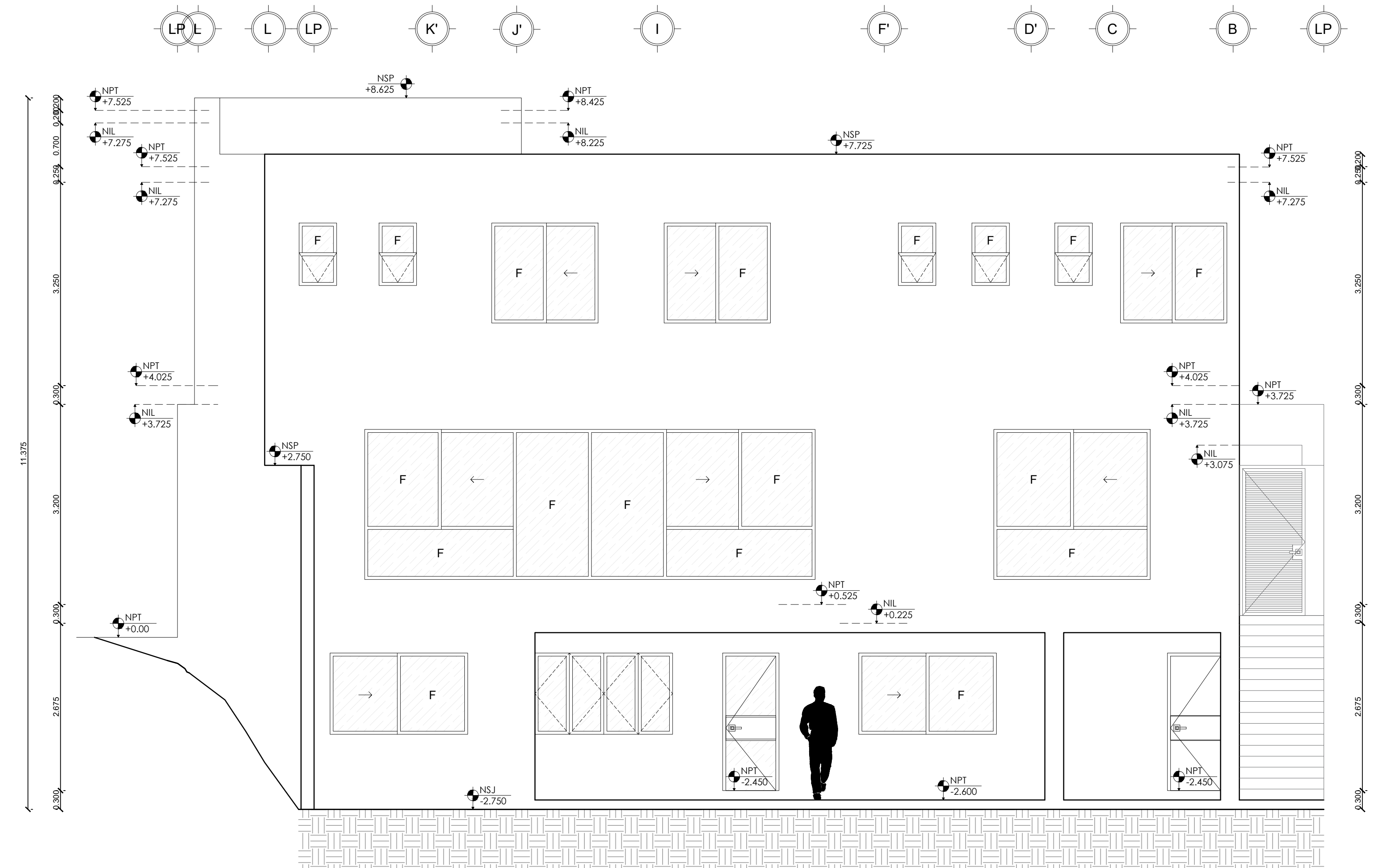
ELEVACION POSTERIOR
