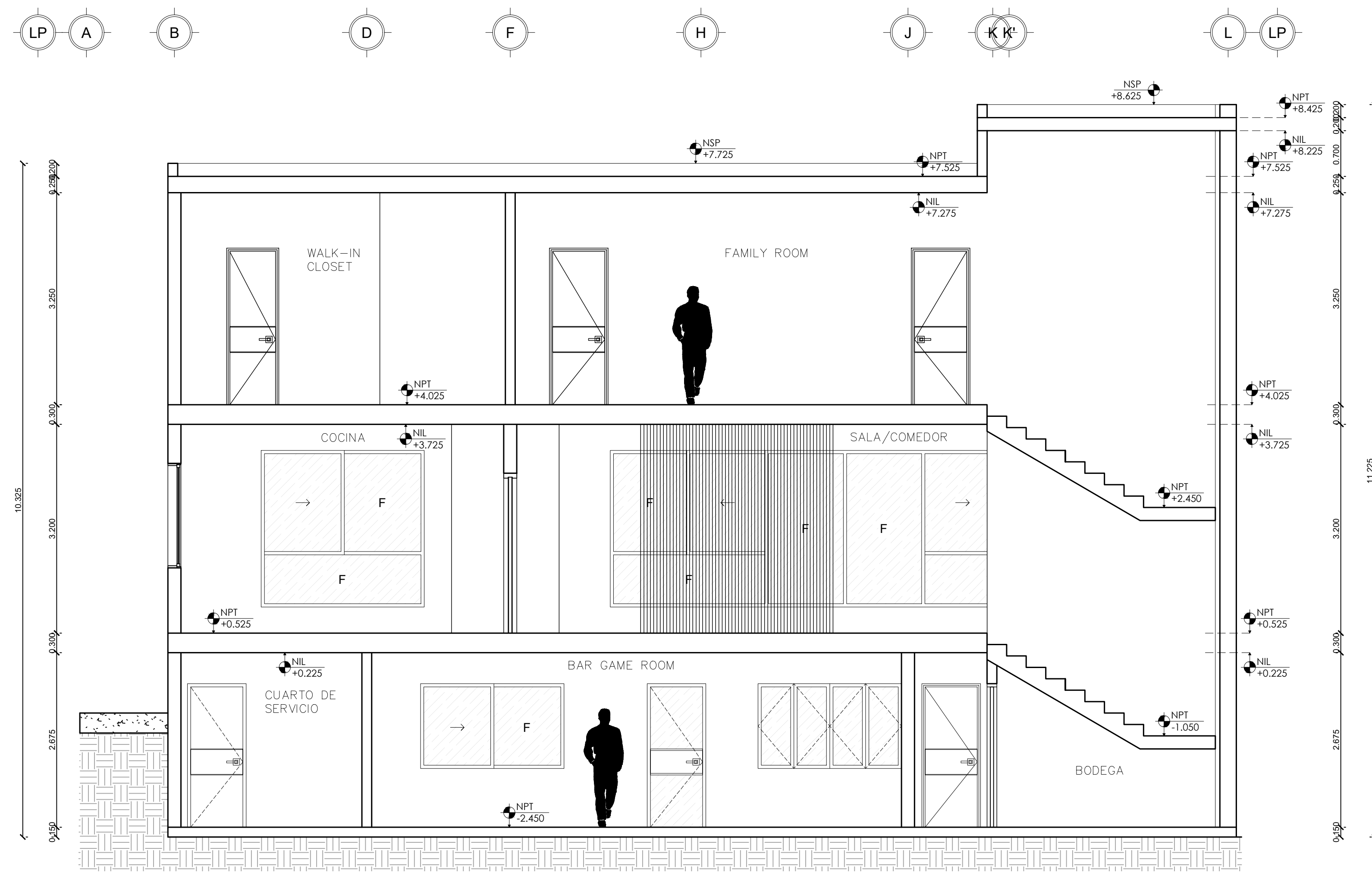
SECCION A-A'
