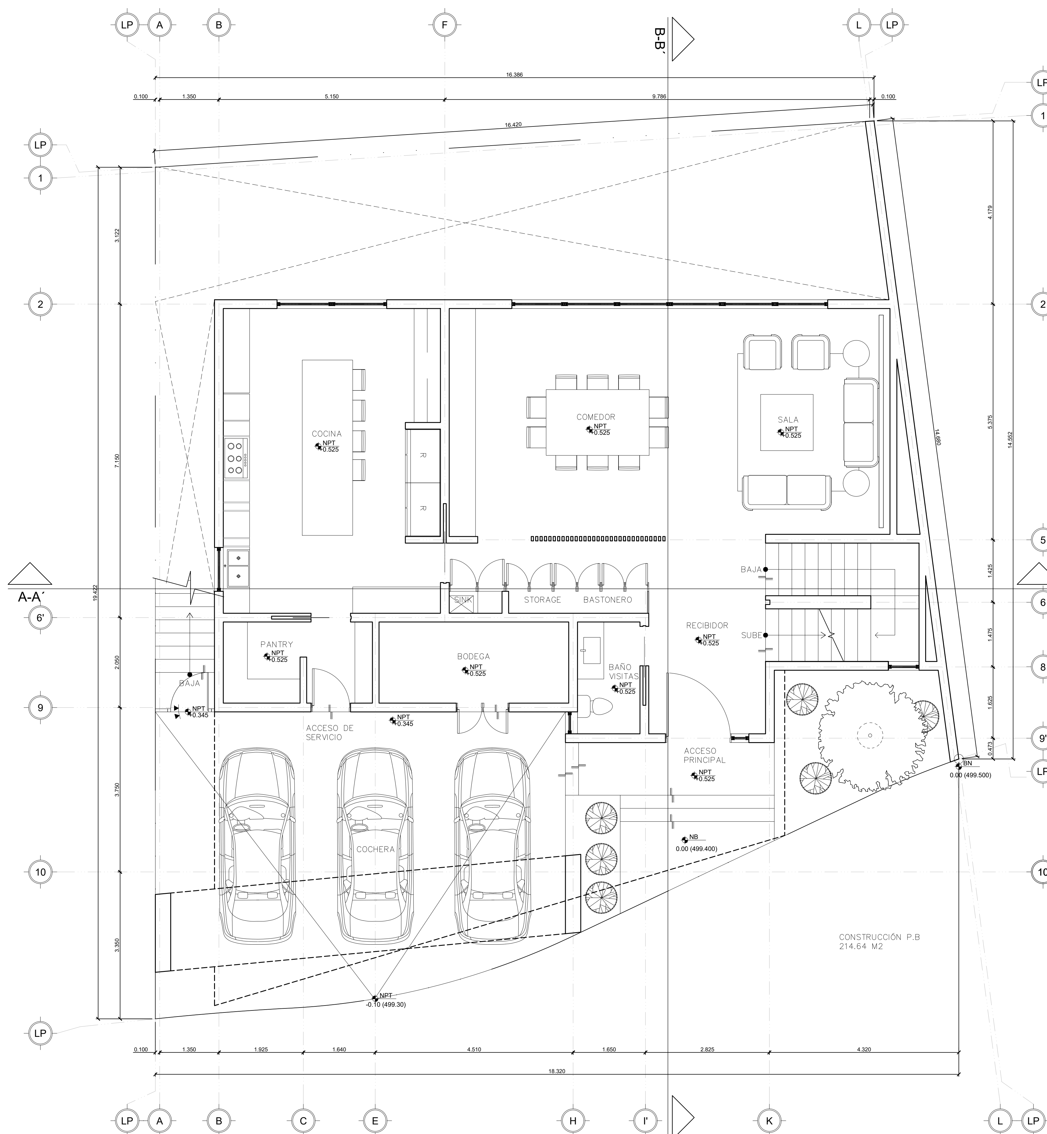
PLANTA BAJA
