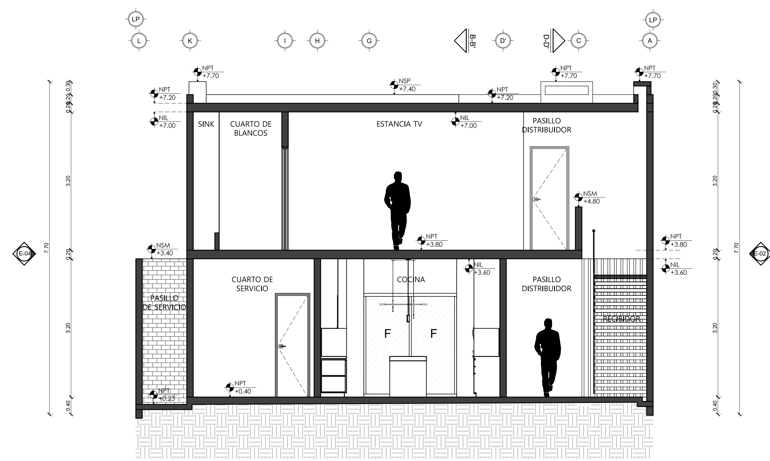
SECCIÓN TRANSVERSAL A-A'
