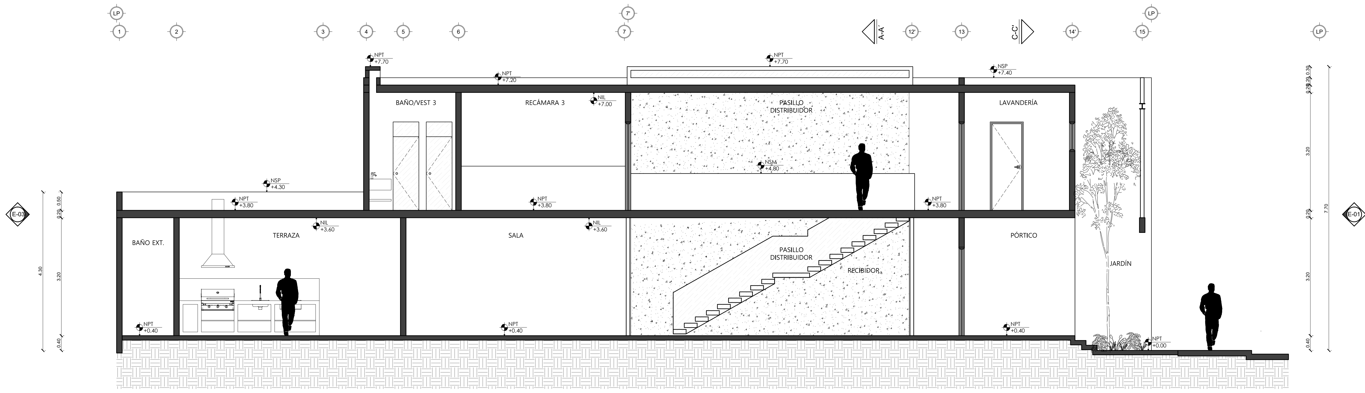
SECCIÓN LONGITUDINAL D-D'
