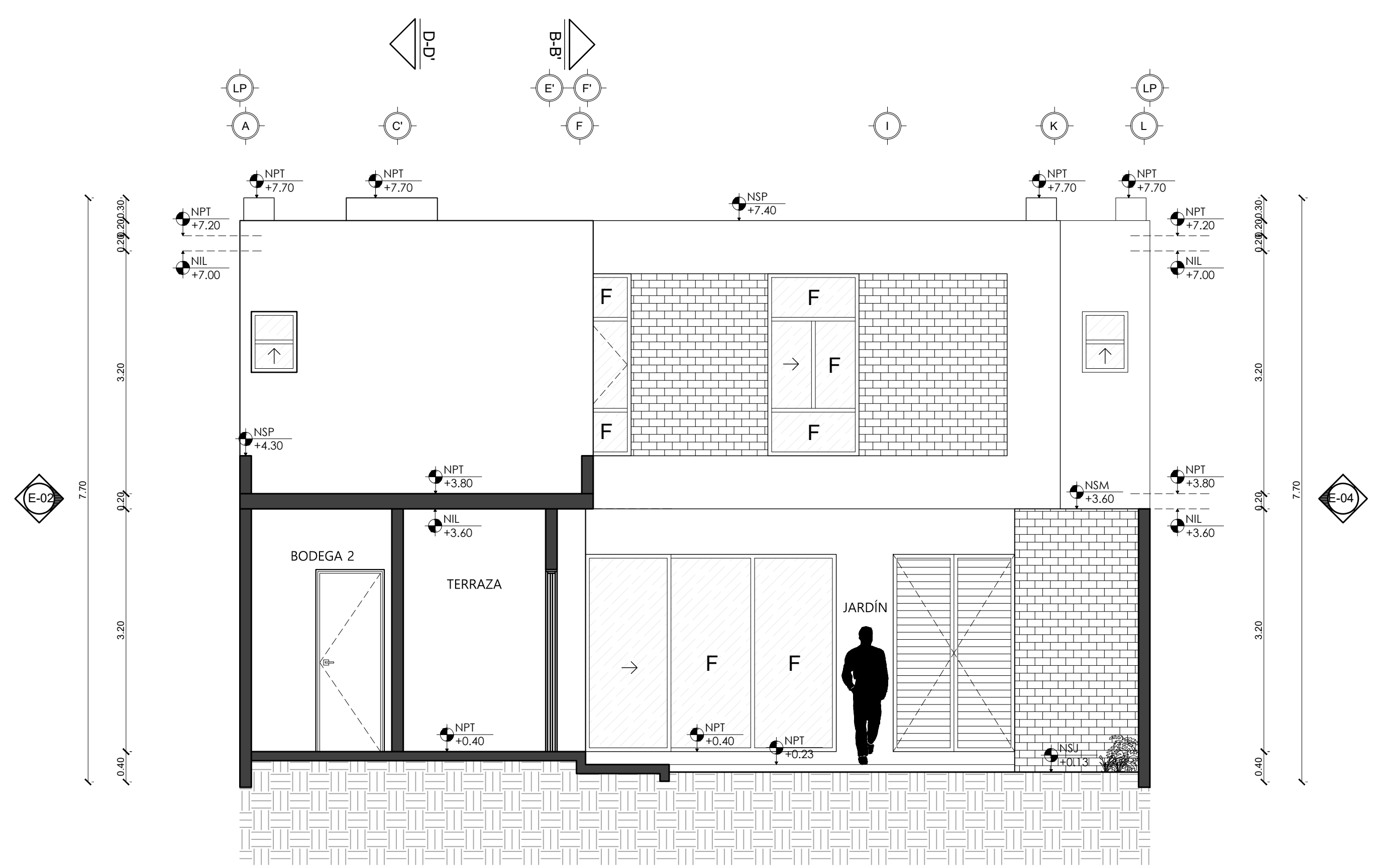
ELEVACIÓN POSTERIOR E-03 (NO)
