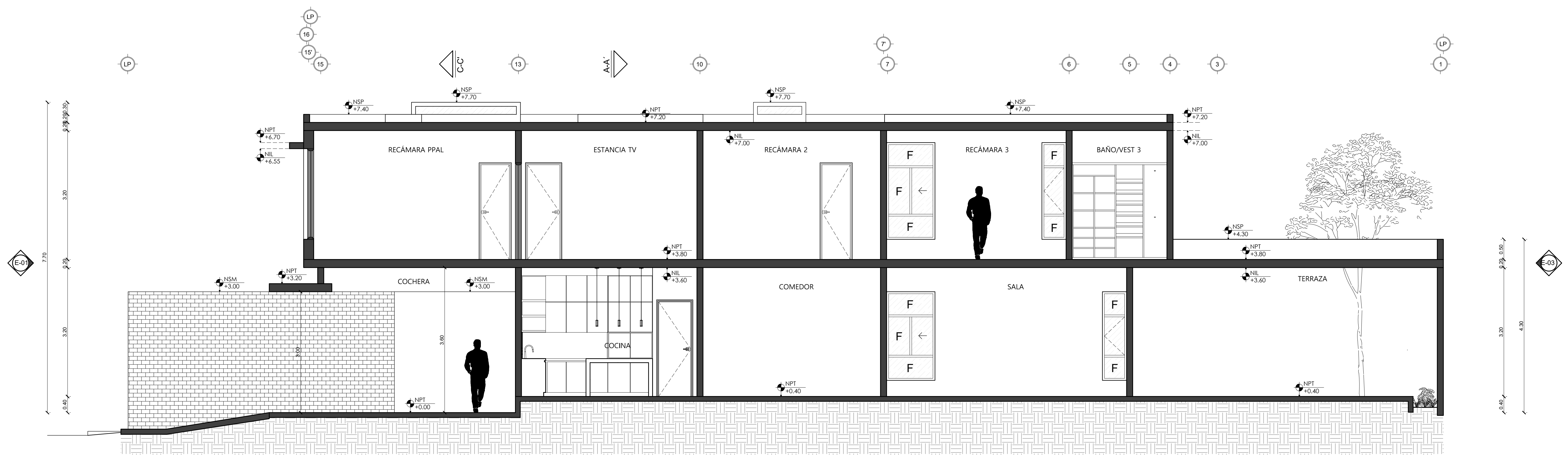
SECCIÓN LONGITUDINAL B-B'
