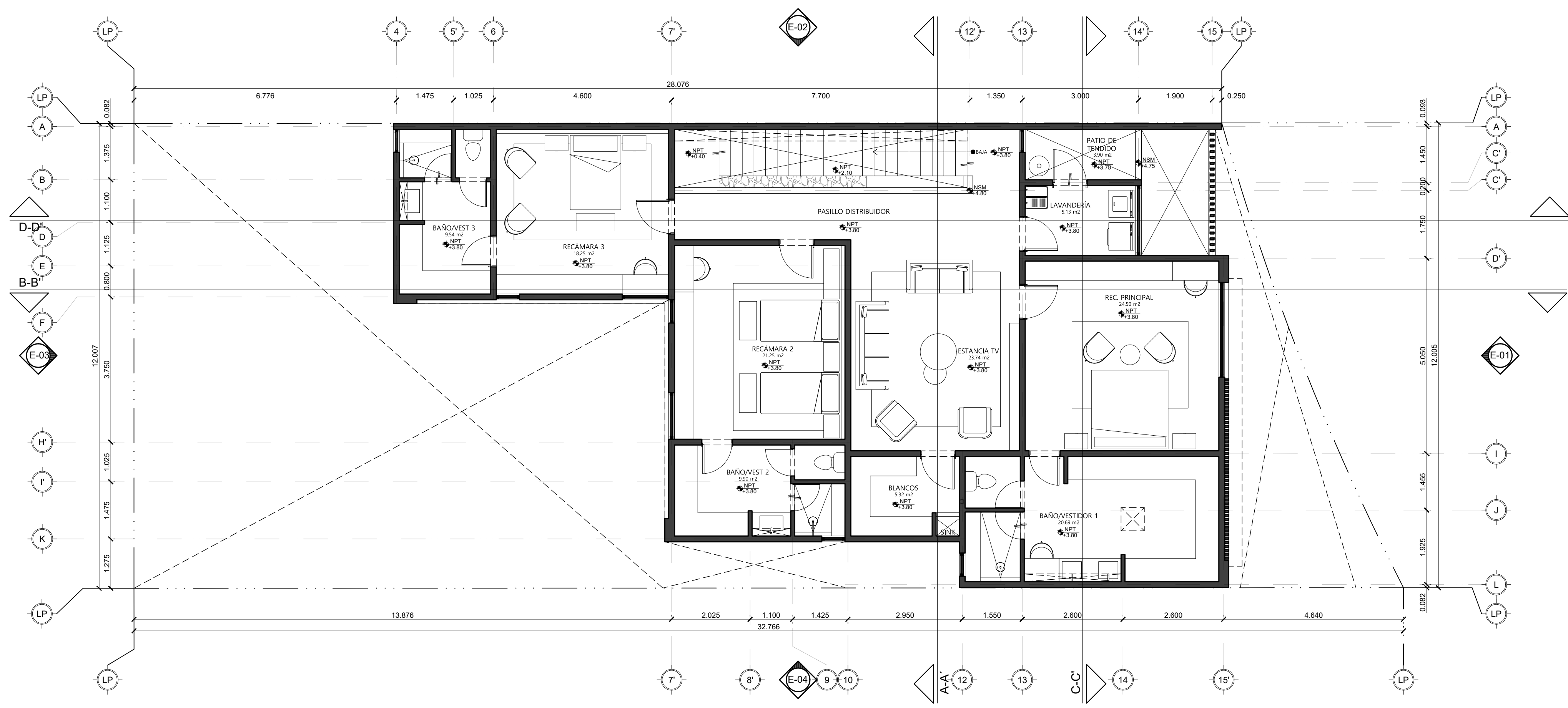
PLANTA ALTA - 188.49 m2
