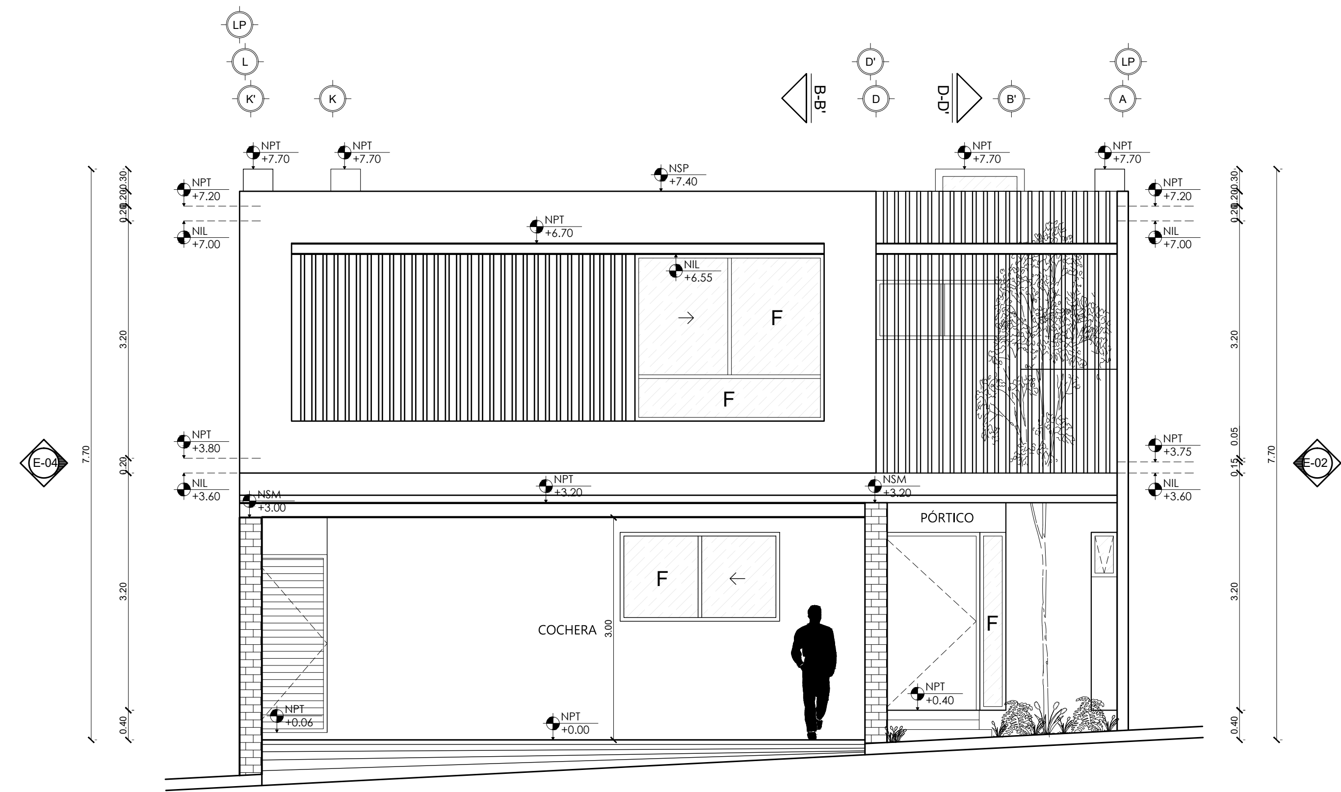
ELEVACIÓN PRINCIPAL E-01 (SE) CASA FÉNIX ESC. 1:50
