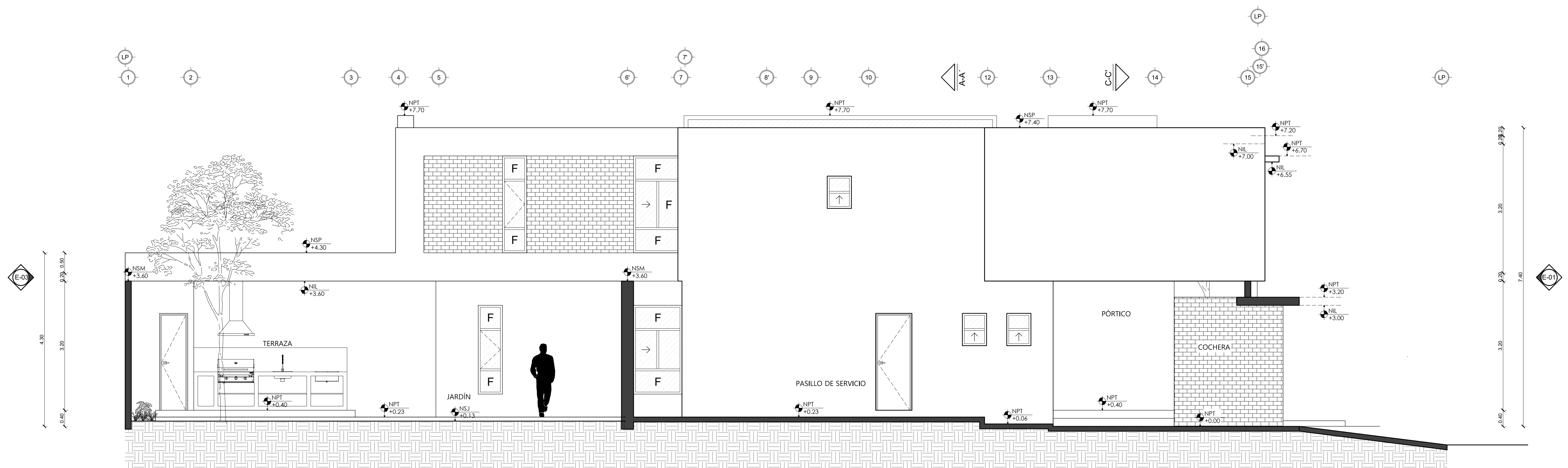
ELEVACIÓN LATERAL IZQUIERDA E-04 (SO)
