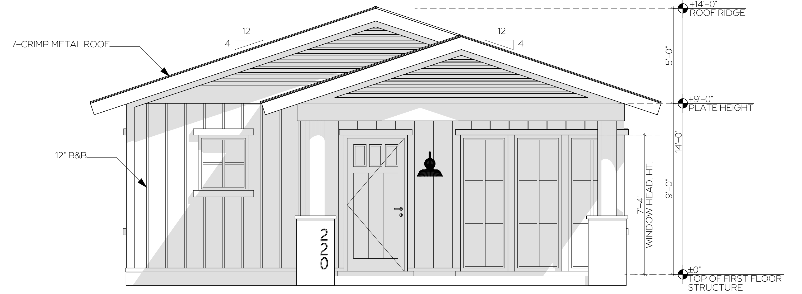
2 A11 FRONT ELEVATION SCALE: 3/8" = 1'-0"
