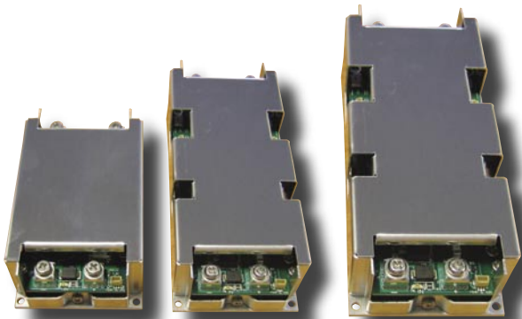
Micro PST14C 150W 100 x 61 x 35mm Mini PST14B 250W 140 x 61 x 35mm Maxi PST14A 500W 225 x 61 x 35mm
