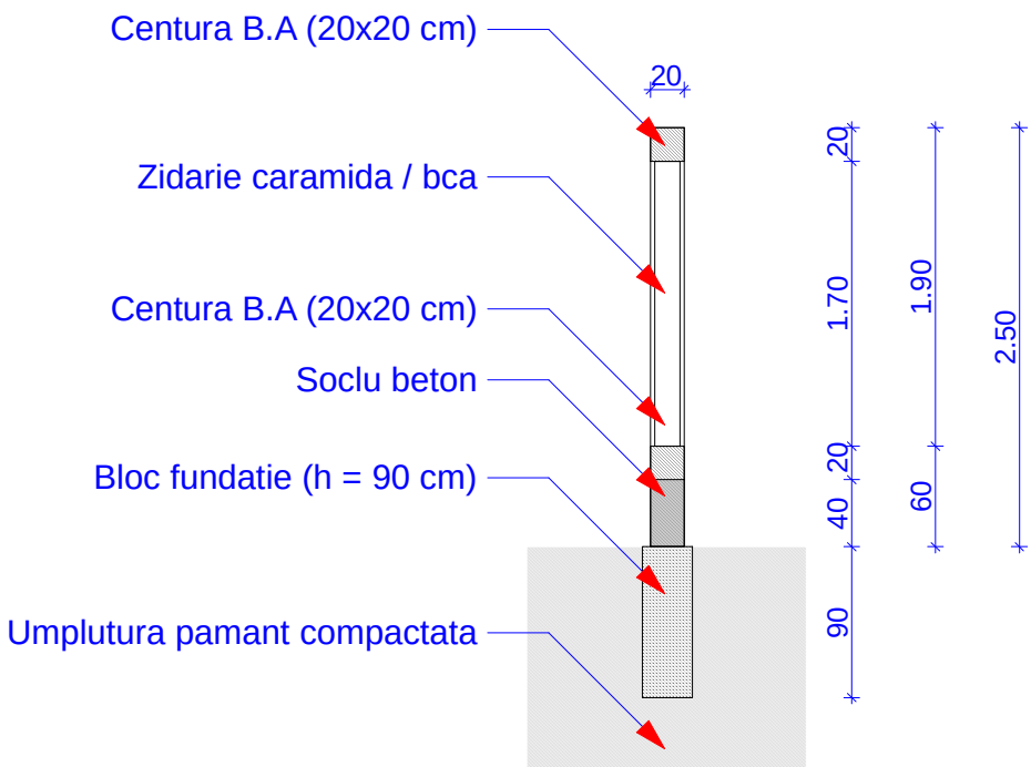
Sectiune
