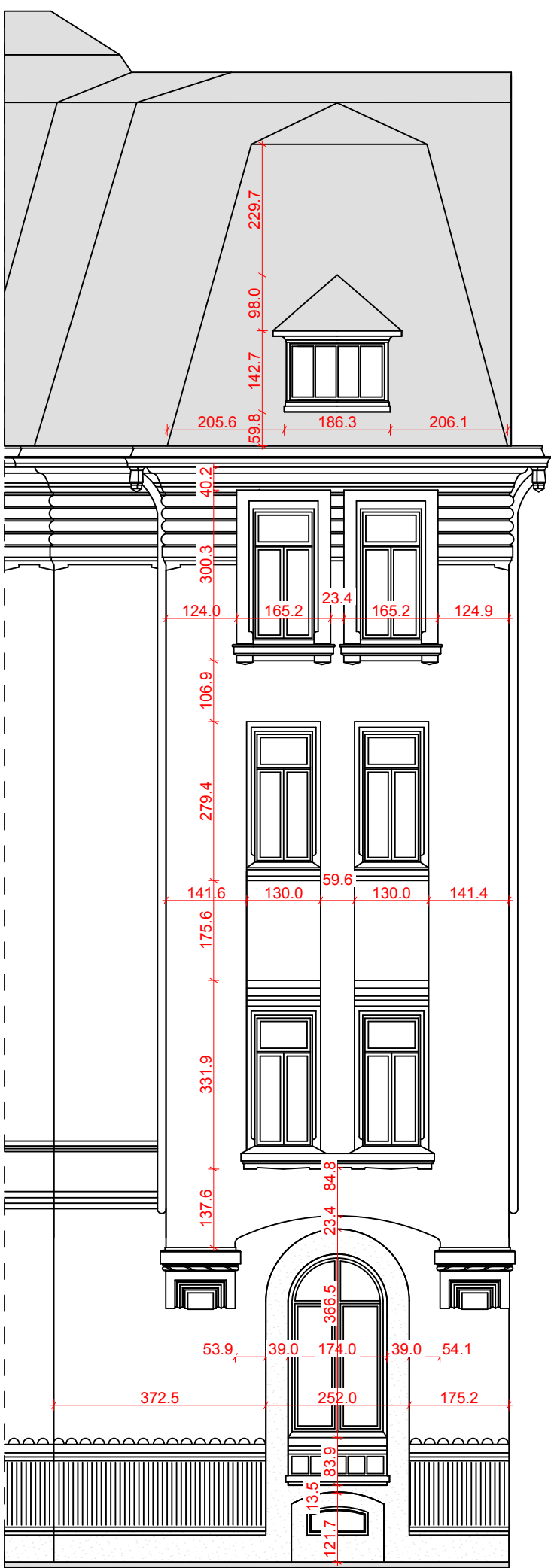
FATADA F.02
