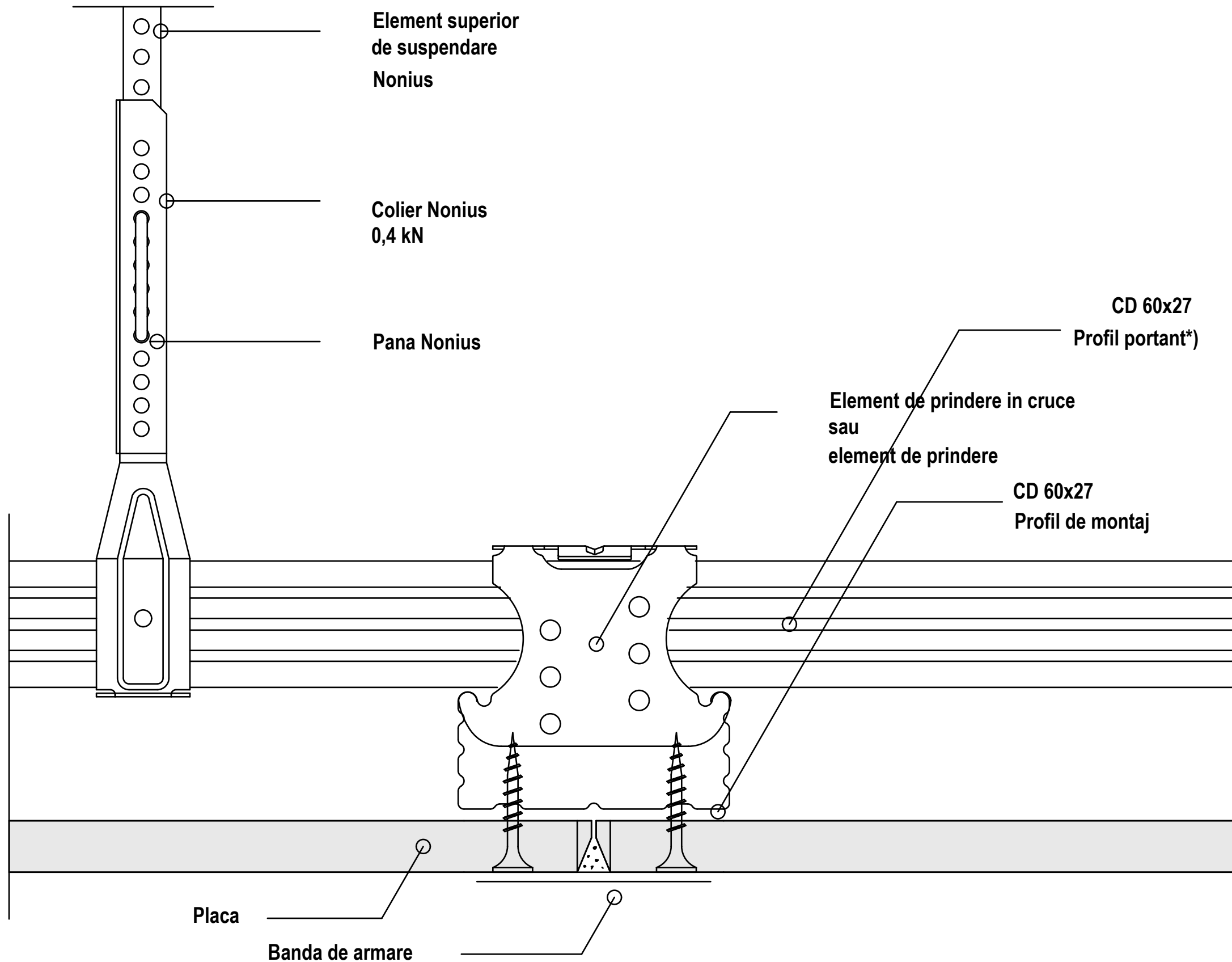
DETALIU TAVAN GIPS CARTON ,IMBINAREA PLACILOR
