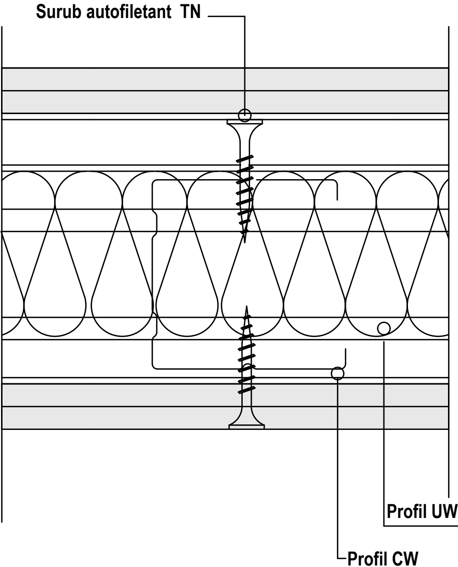
DETALIU PERETE GIPS CARTON,IMBINAREA PLACILOR
