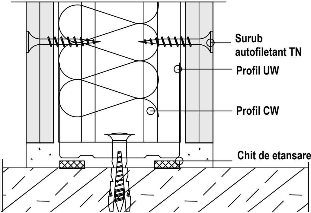
DETALIU PERETE GIPS CARTON,SECTIUNE VERTICALA
