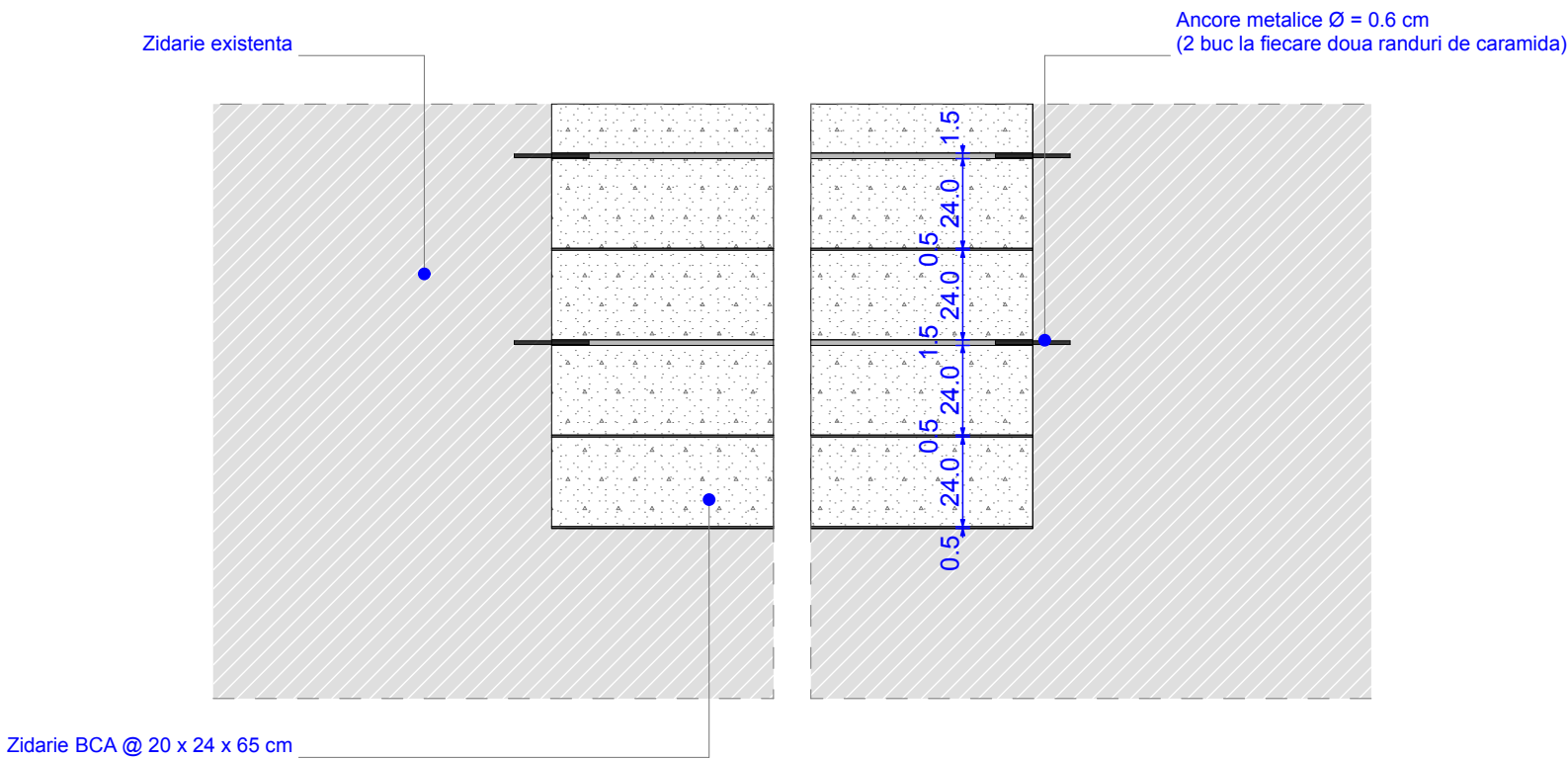
SECTIUNE LONGITUDINALA
