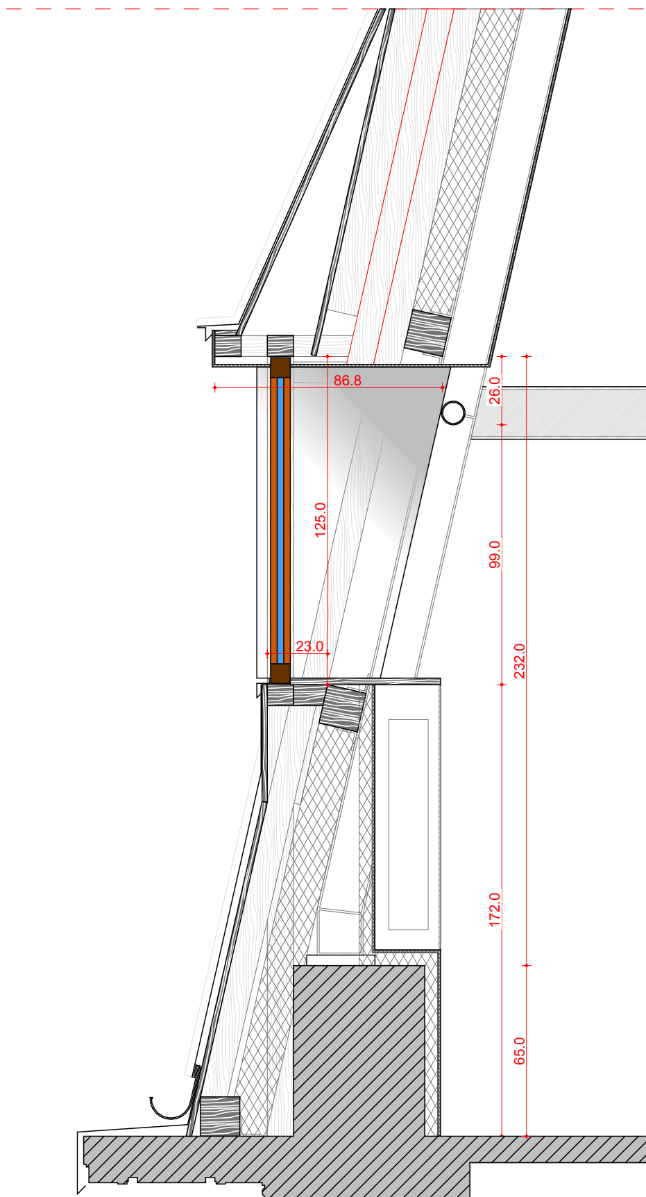
SECTIONE
