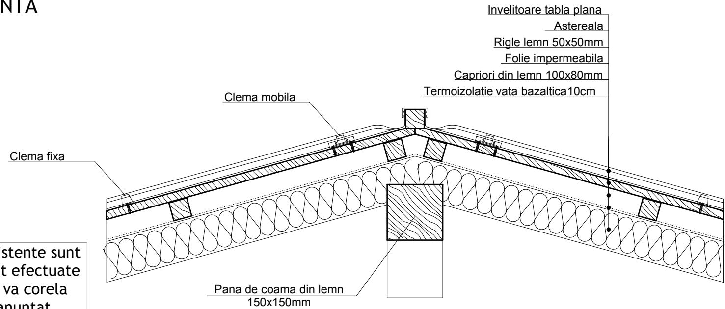
DETALIU PANA DE COAMA
