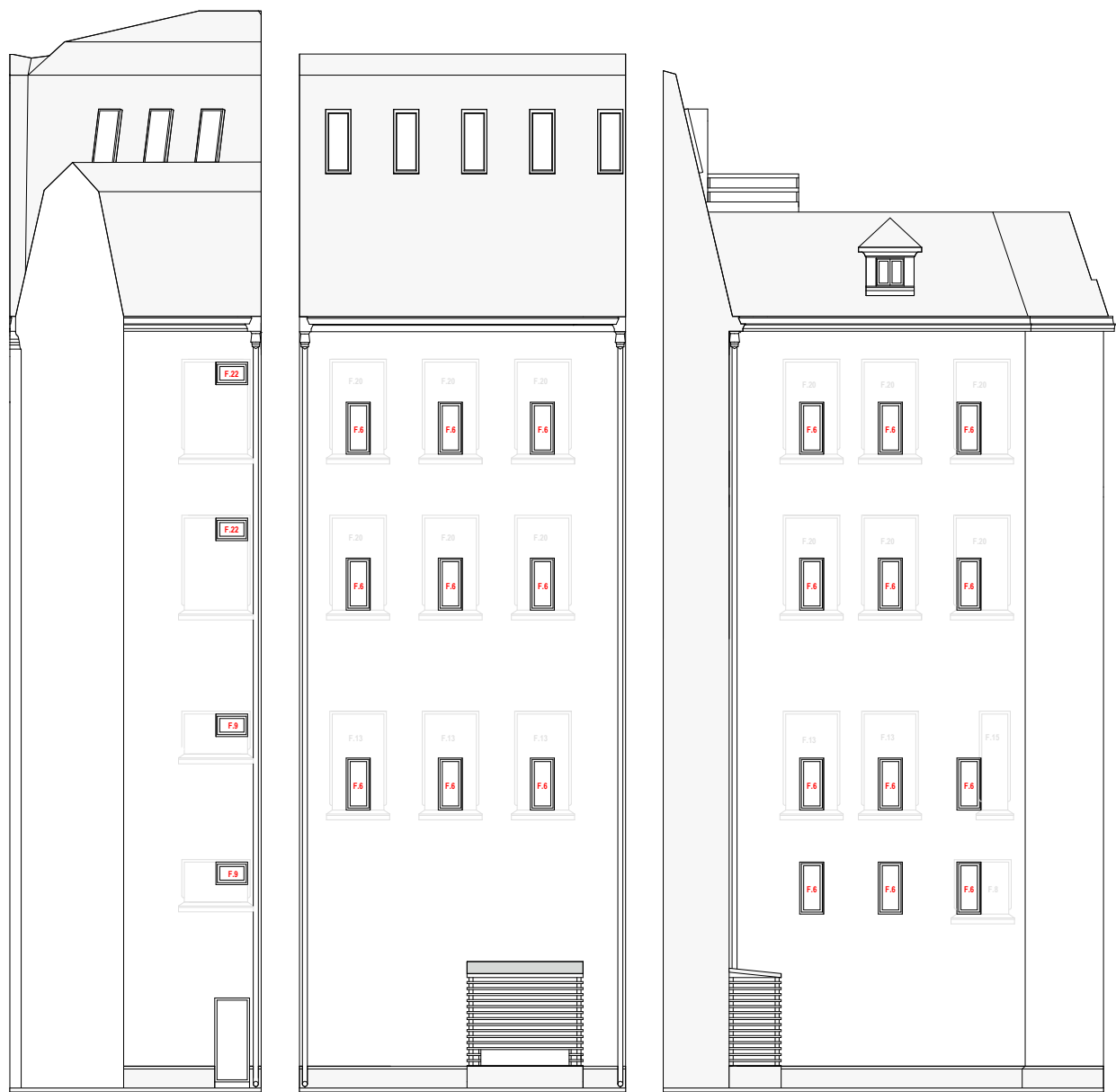
FATADA F.07
