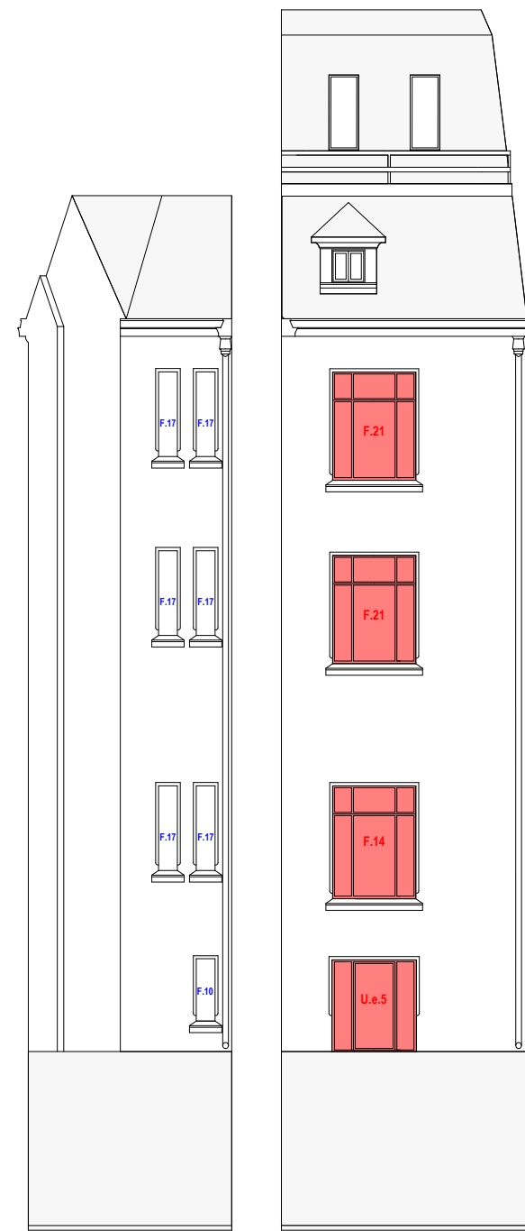
FATADA F.10
