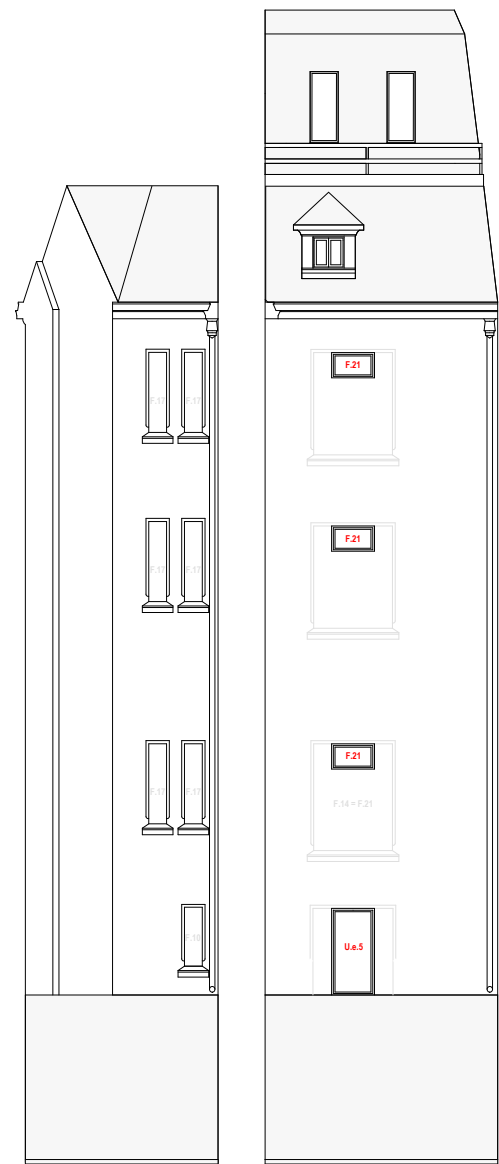
FATADA F.10
