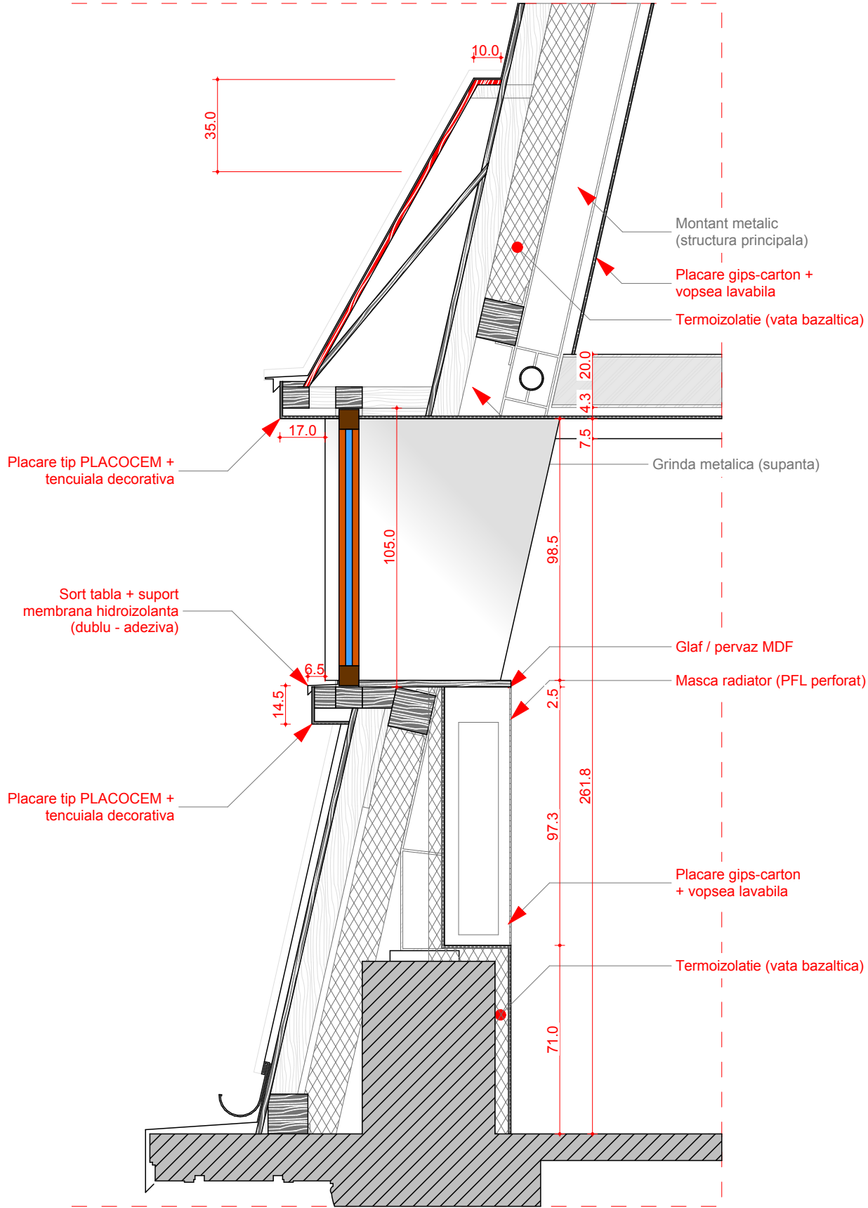
SECTIUNE
