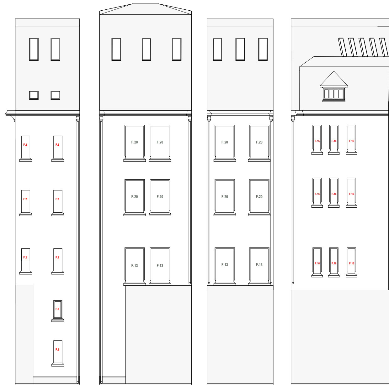
FATADA F.03
