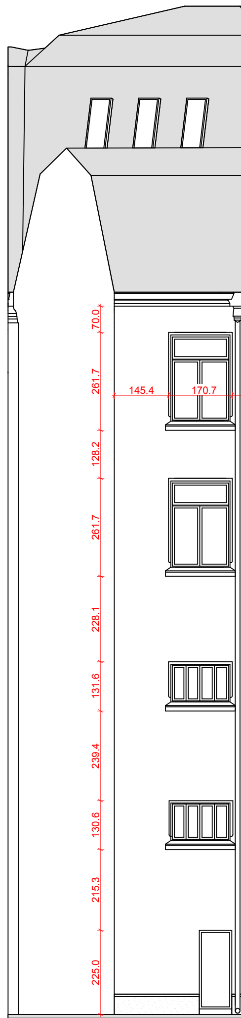
FATADA F.07
