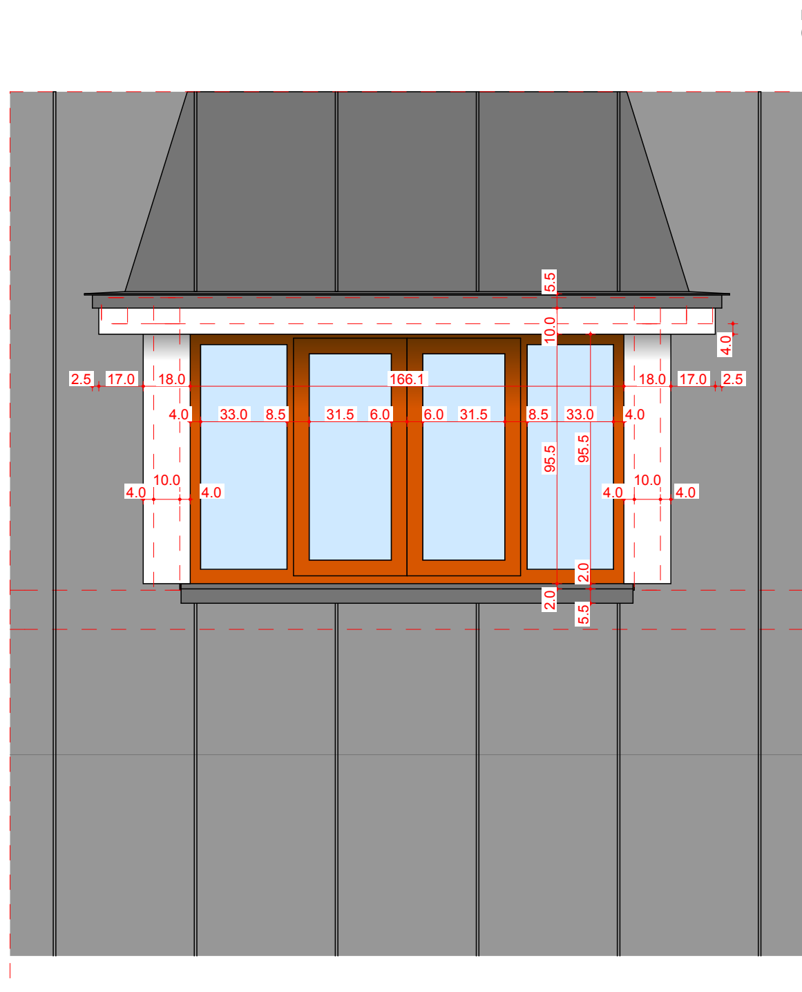
VEDERE EXTERIOARA
