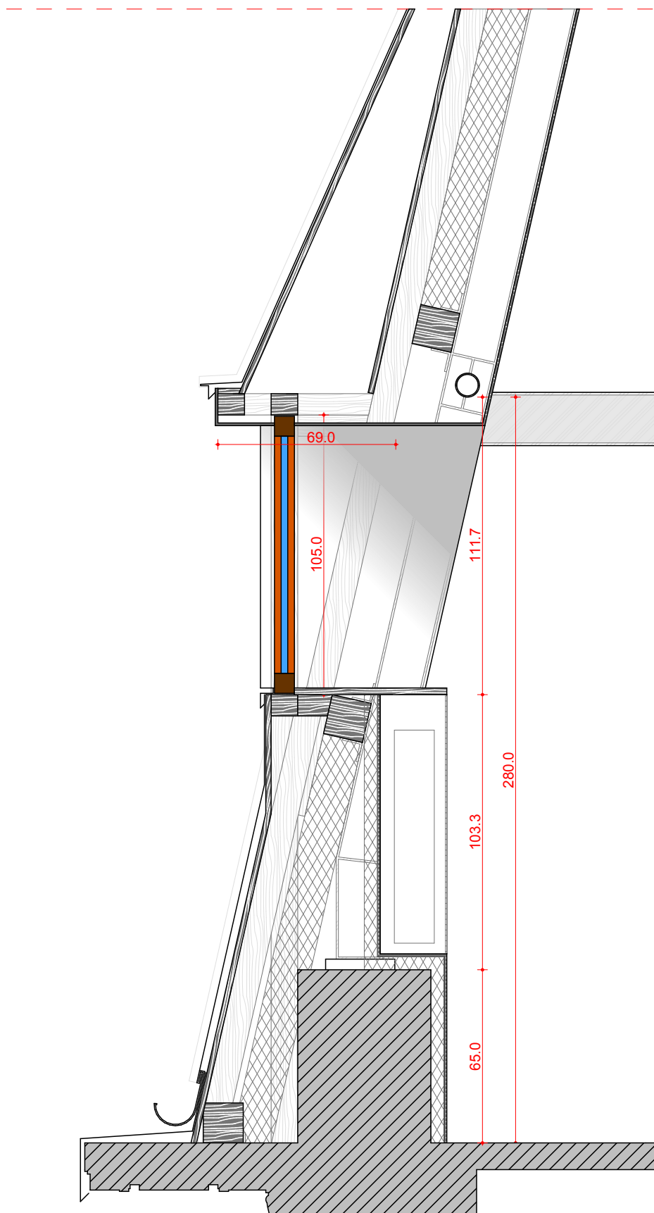
SECȚIUNE
