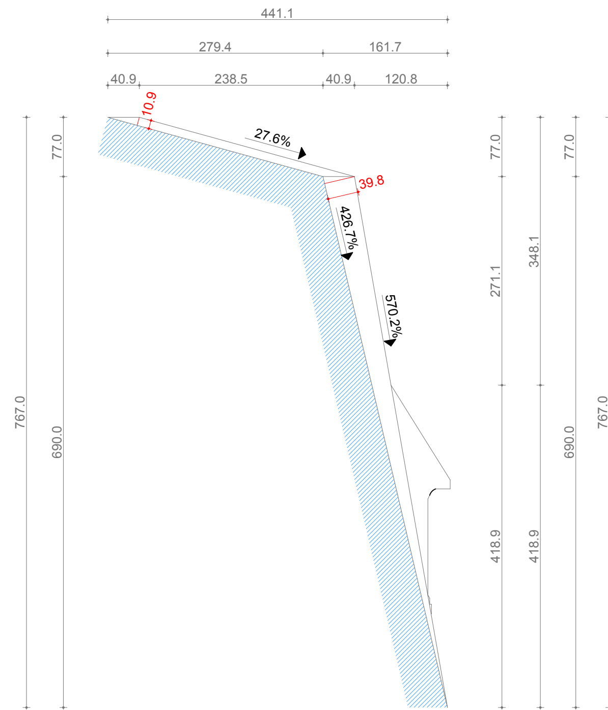
SECTIUNE - ACOPERIS (zona colt) (var. 1 - initiala la ~ 41 cm)
