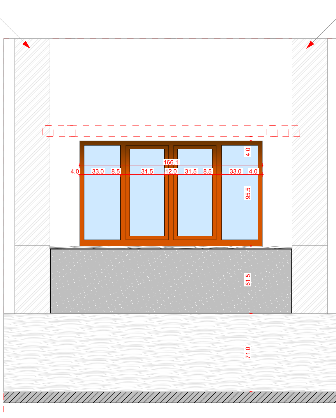
VEDERE INTERIOARA
