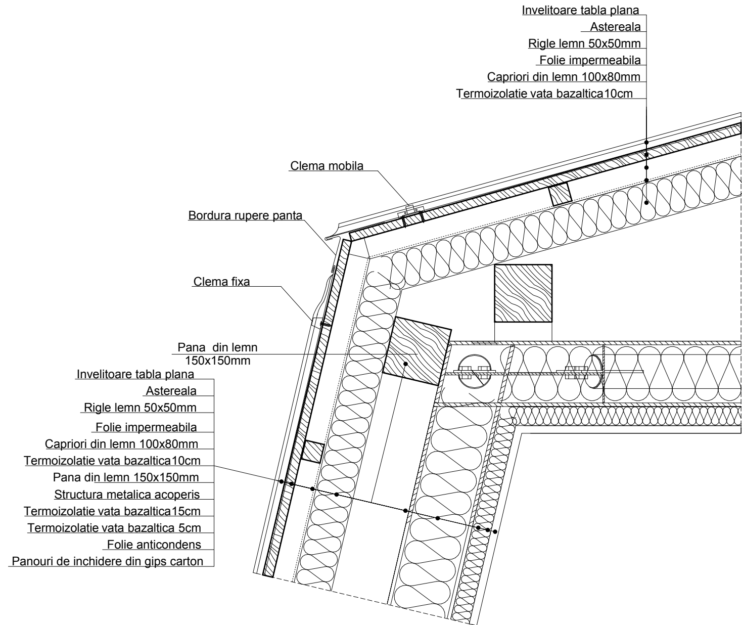
DETALIU RUPERE DE PANTA
