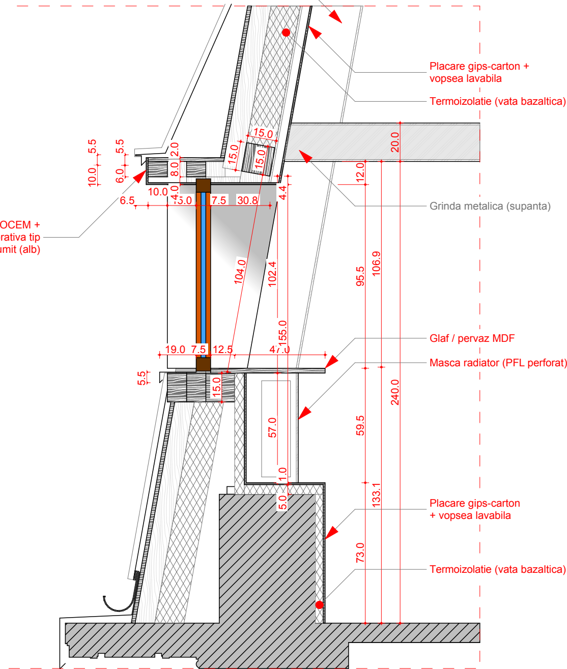
SECTIUNE
