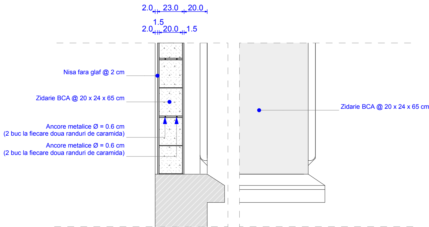
SECTIUNE TRANSVERSALA
