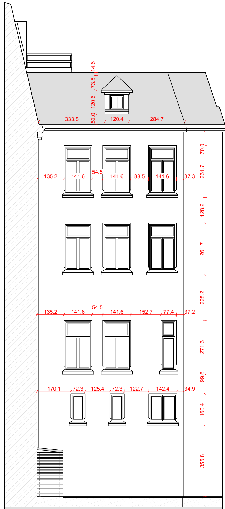
FATADA F.09
