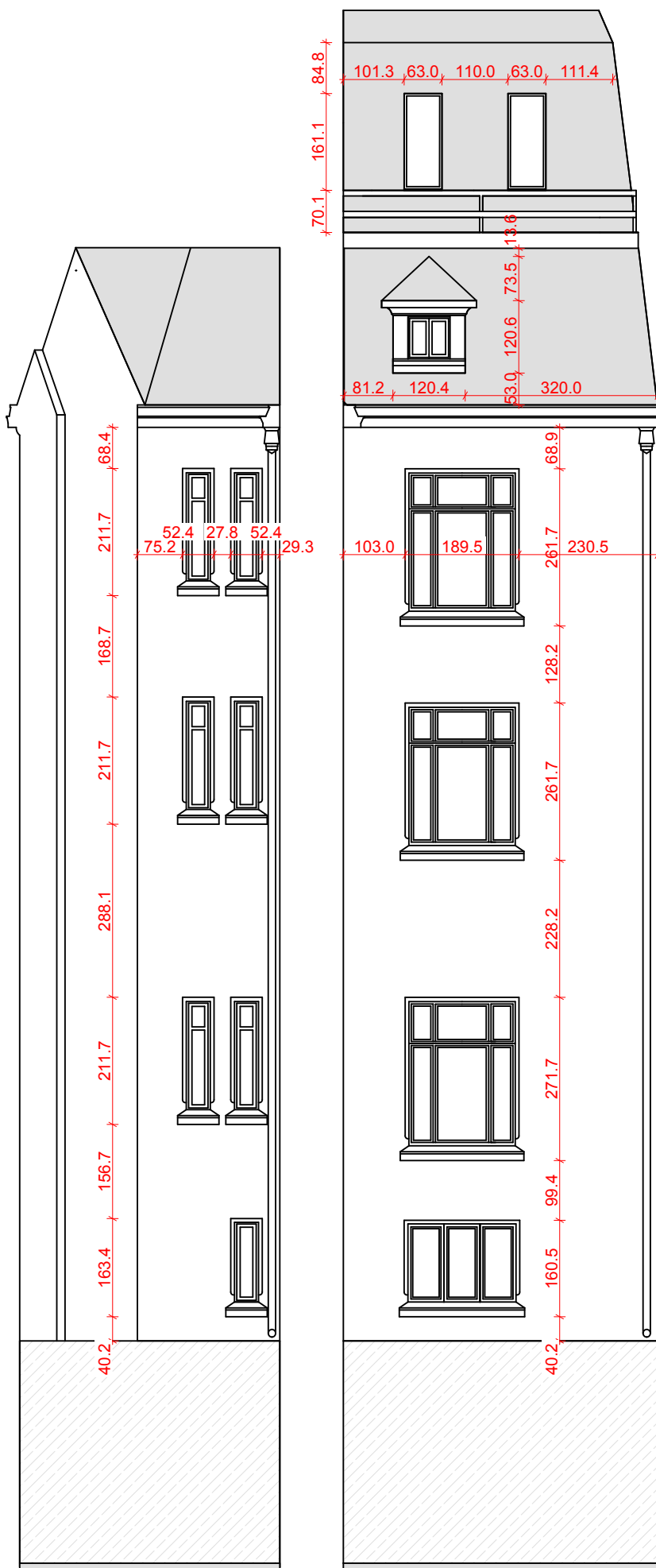
FATADA F.10
