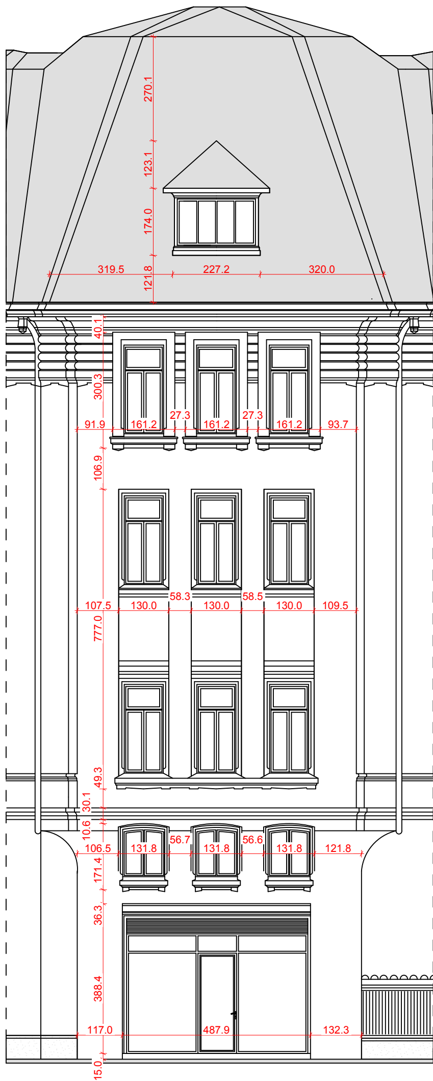
FATADA F.01
