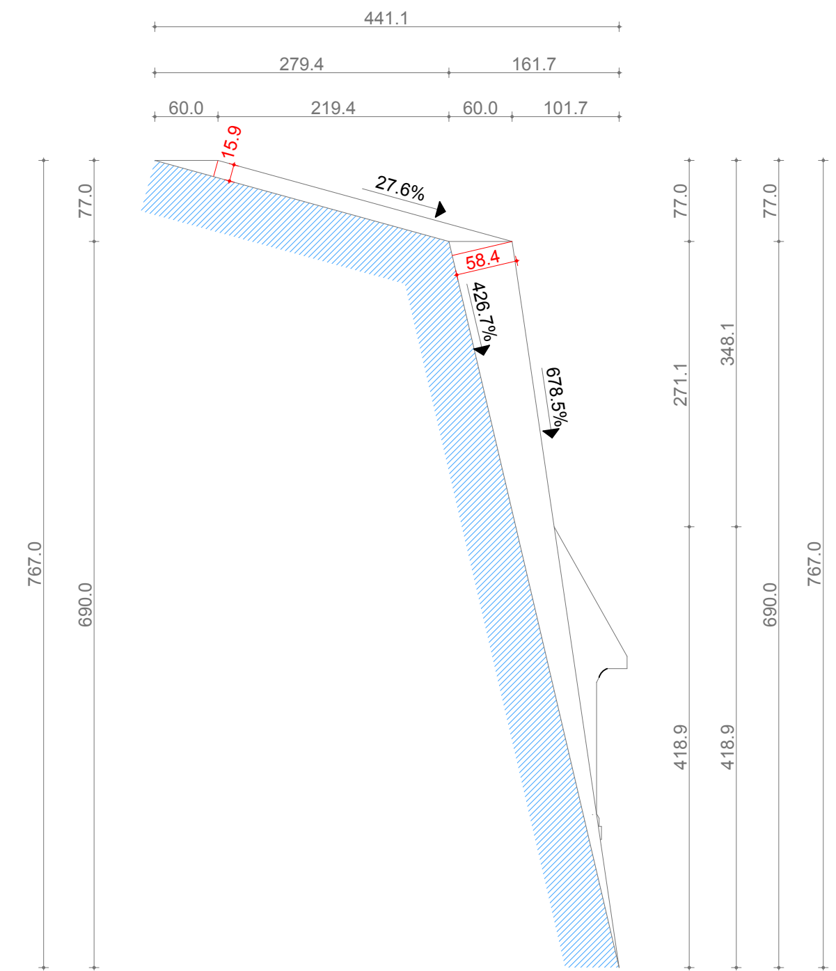
SECTIUNE - ACOPERIS (zona colt) (var. 2 - extinsa la 60 cm)
