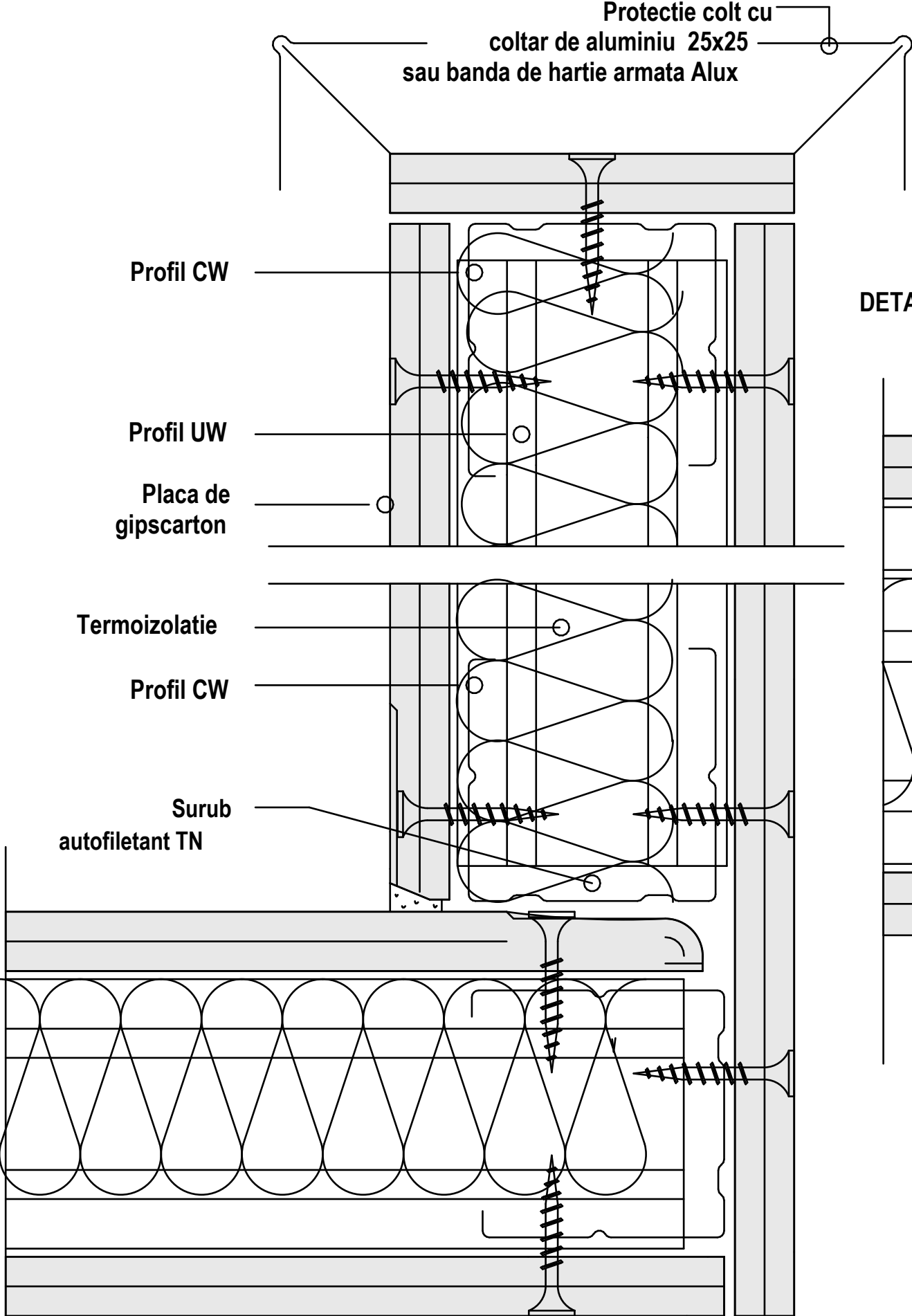
DETALIU PERETE GIPS CARTON,REALIZAREA COLTURILOR
