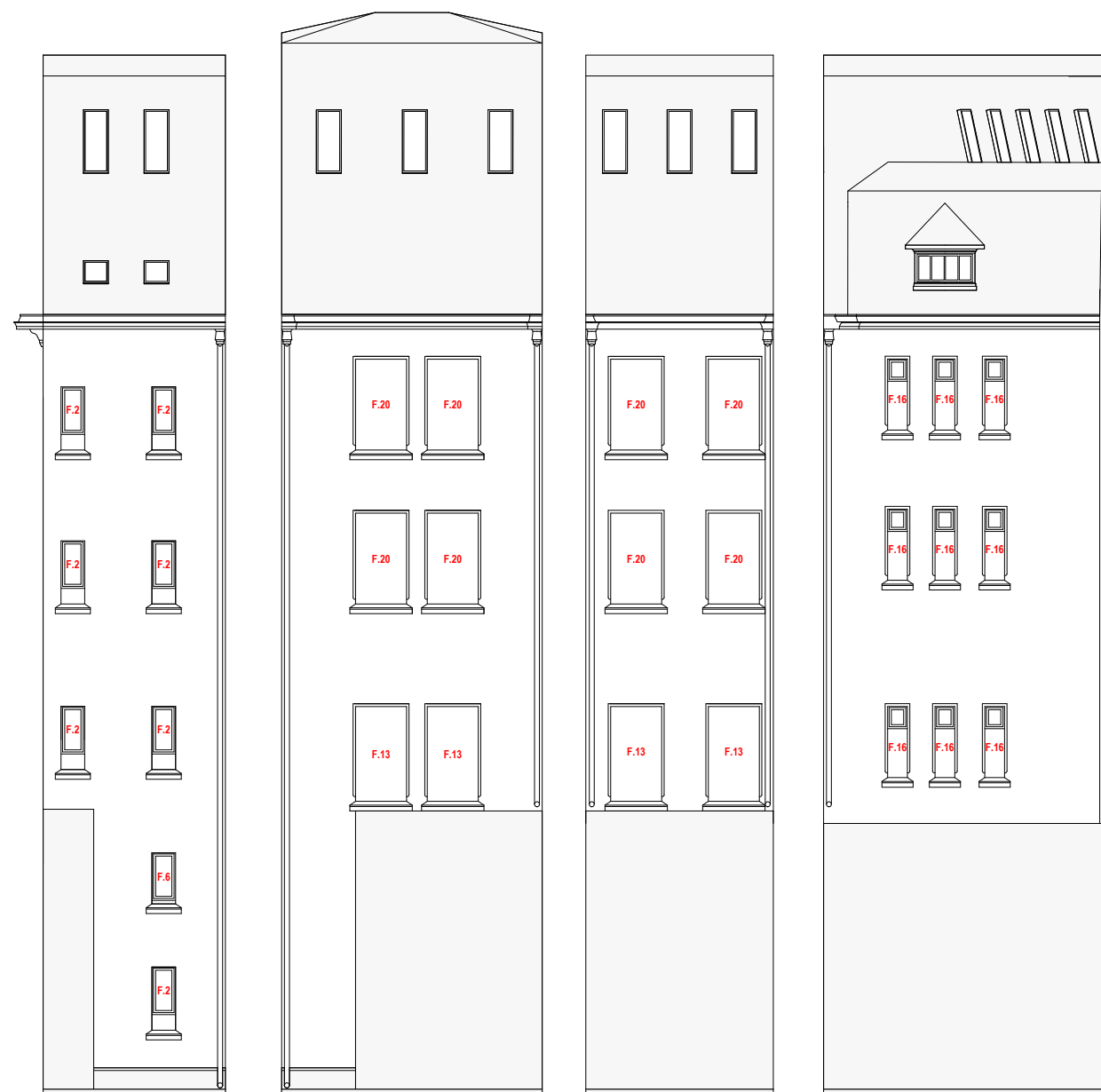
FATADA F.03
