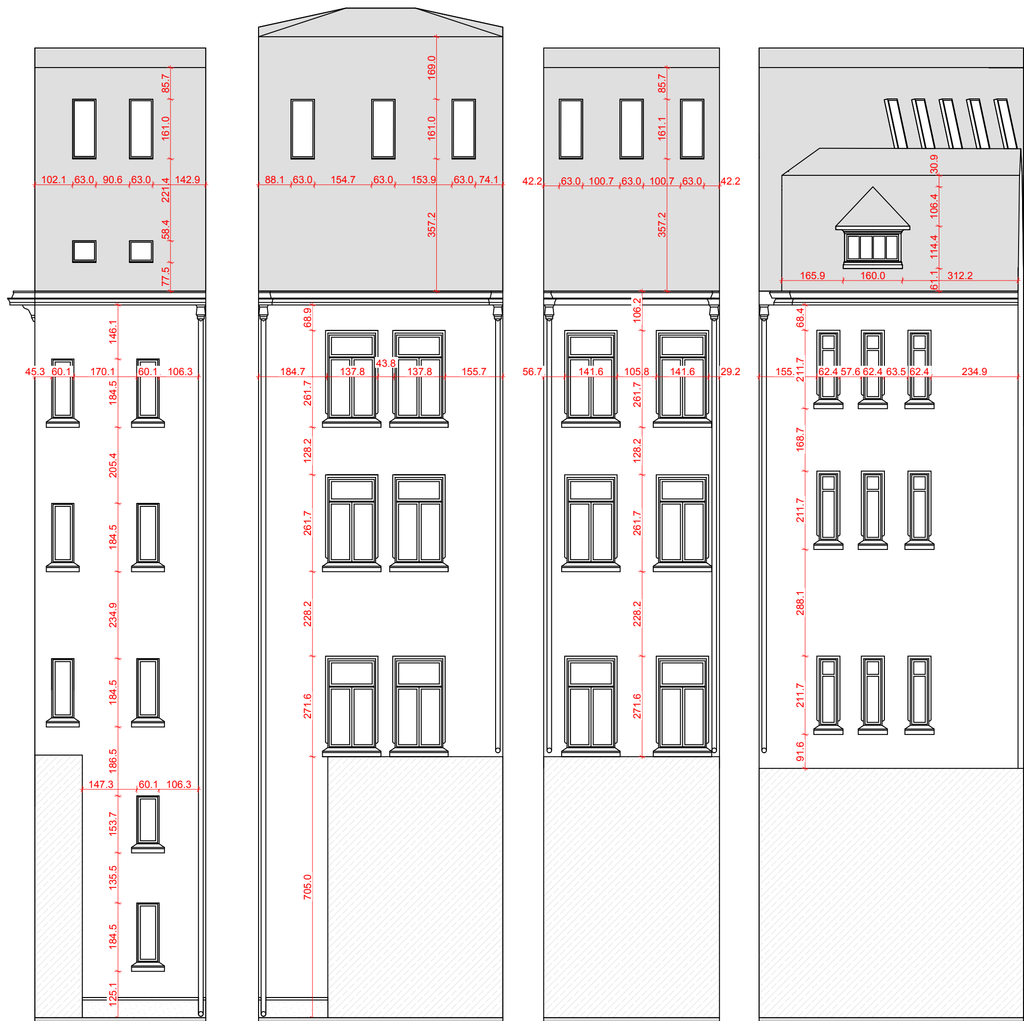
FATADA F.03
