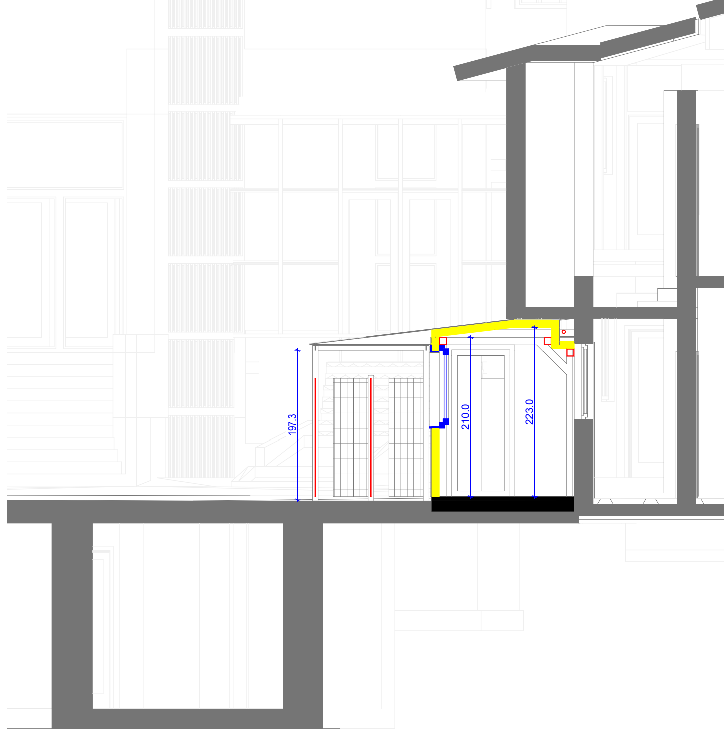
SECTIONE TRANSVERSALA
