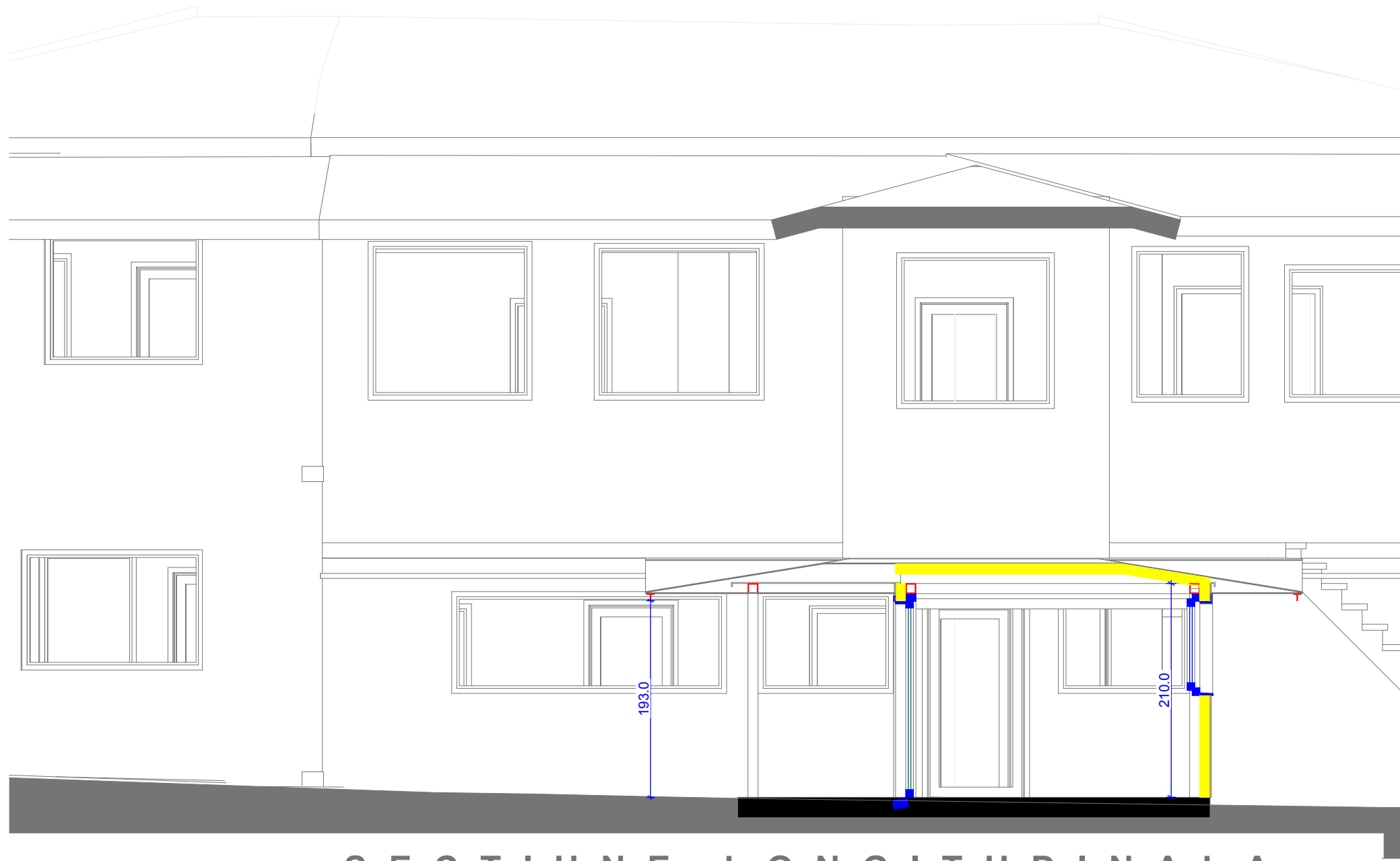
SECTIONE LONGITUDINALA
