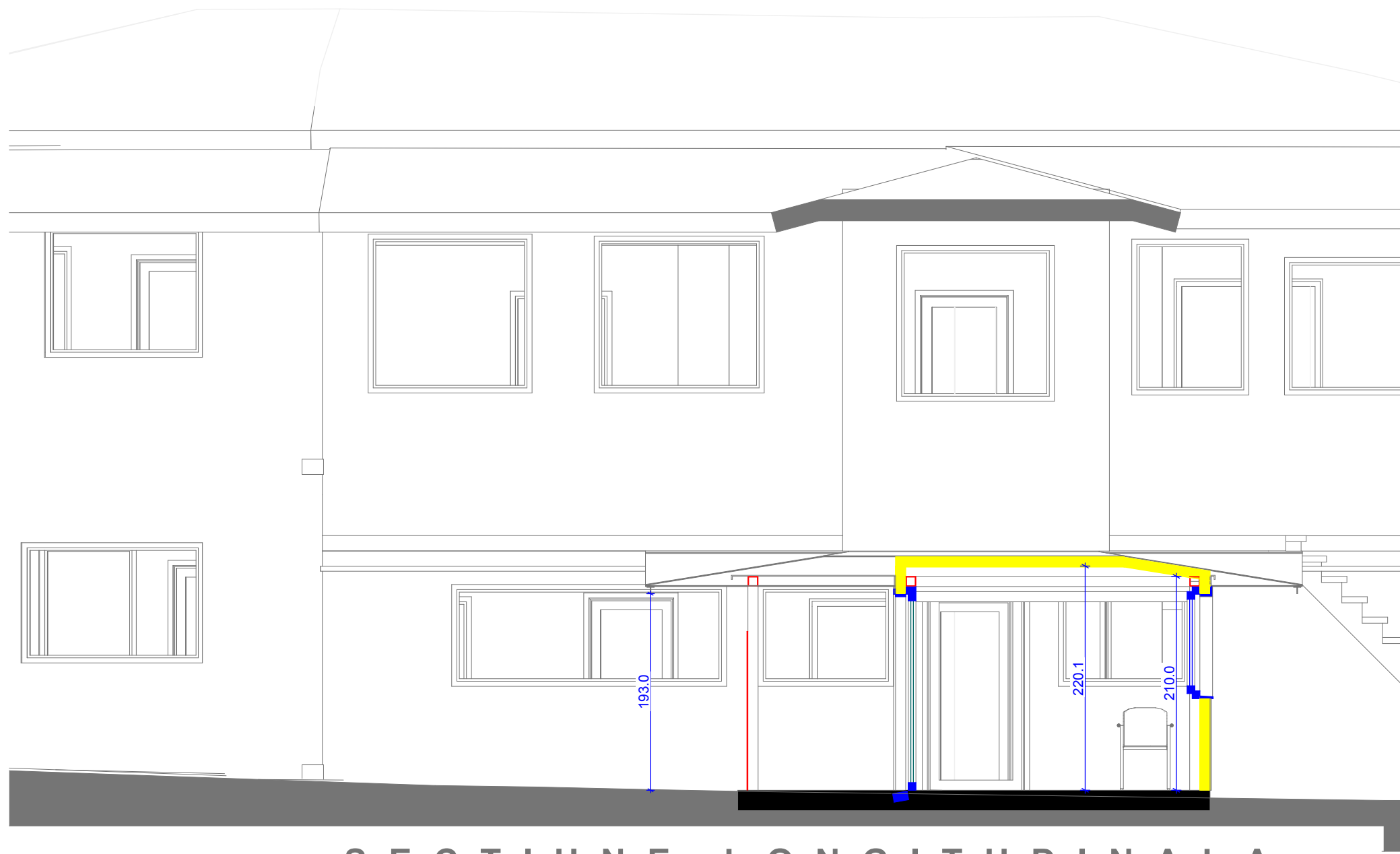
SECTIUNE LONGITUDINALA
