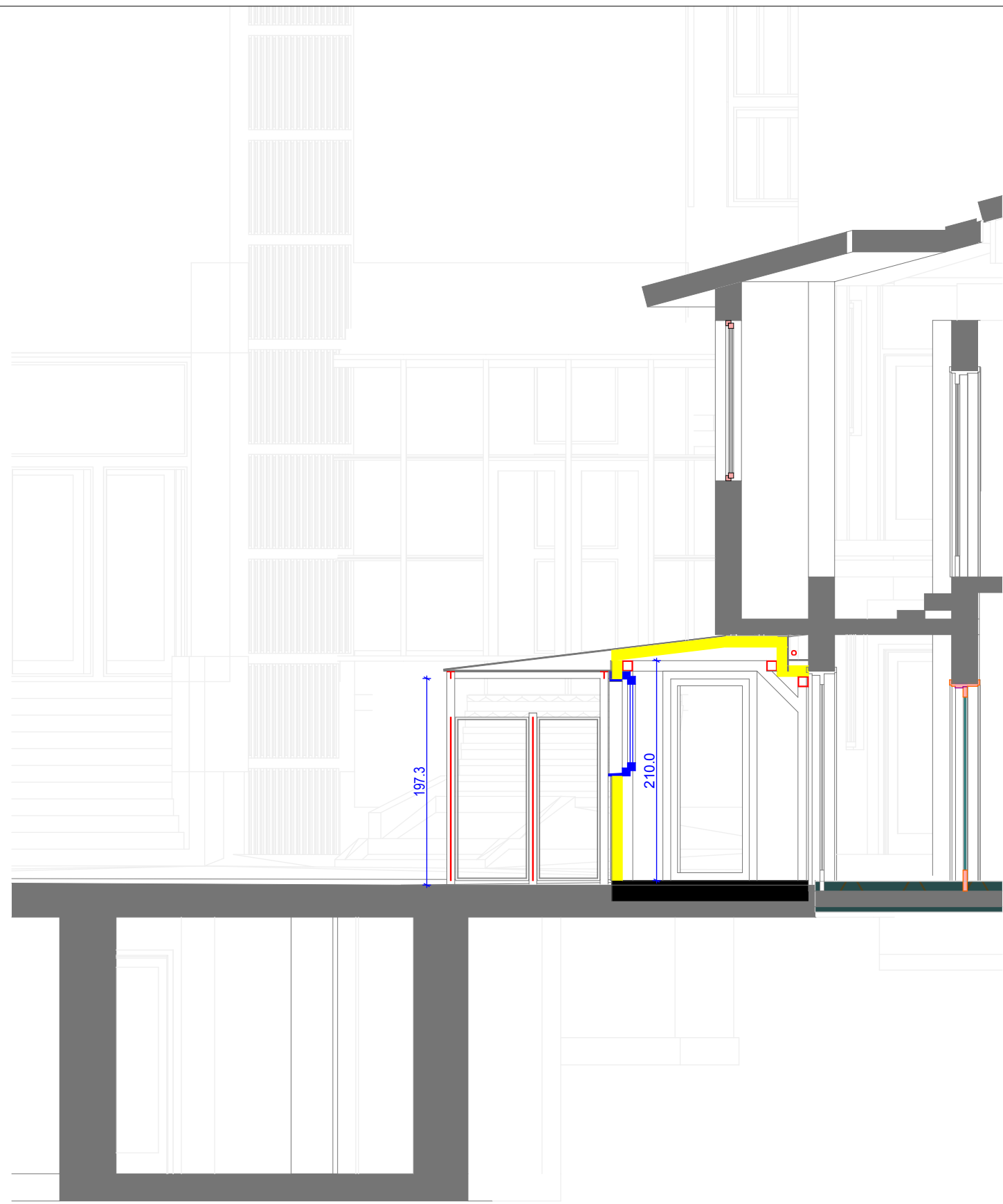
S E C T I U N E T R A N S V E R S A L A
