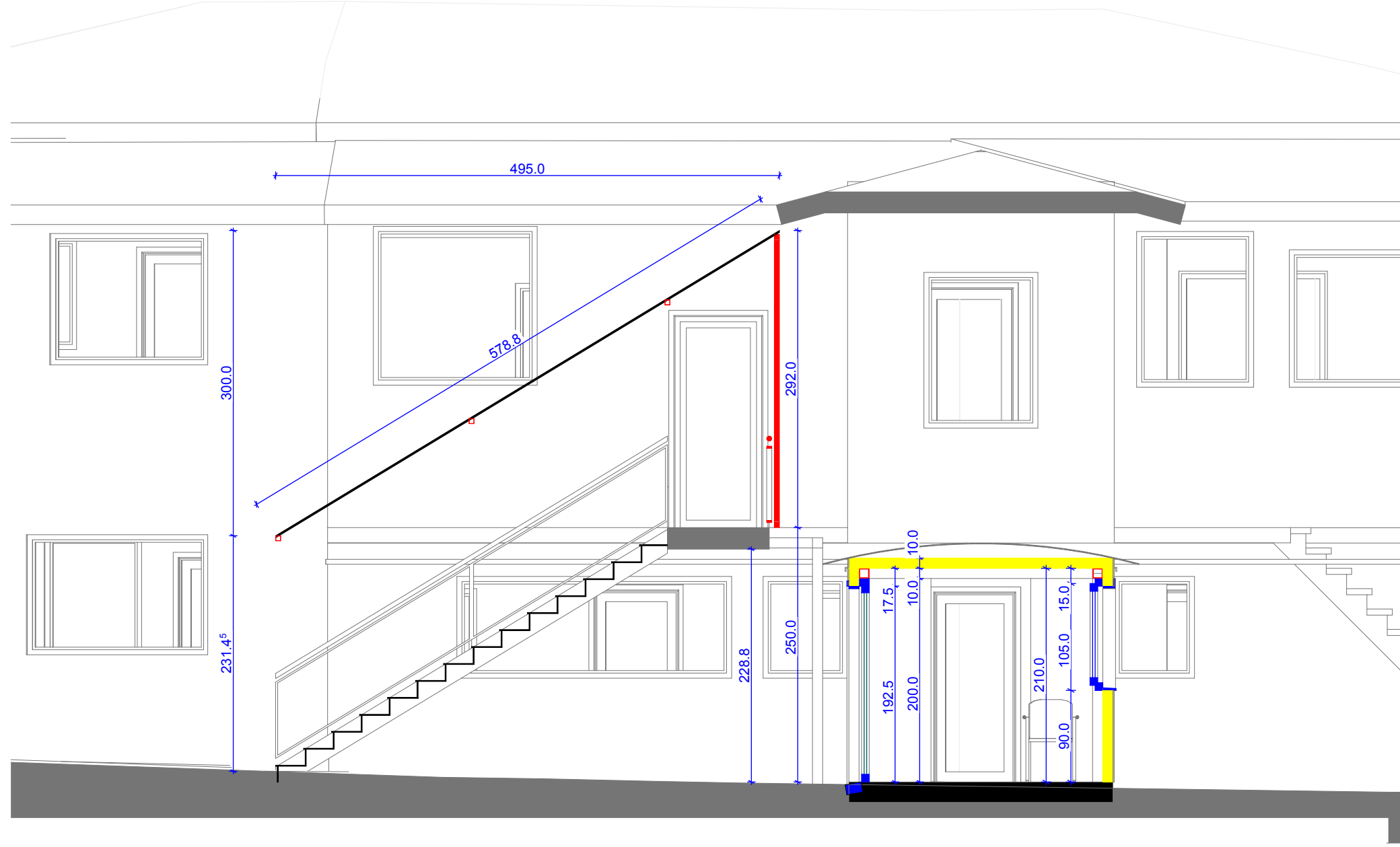
S E C T I O N E A
