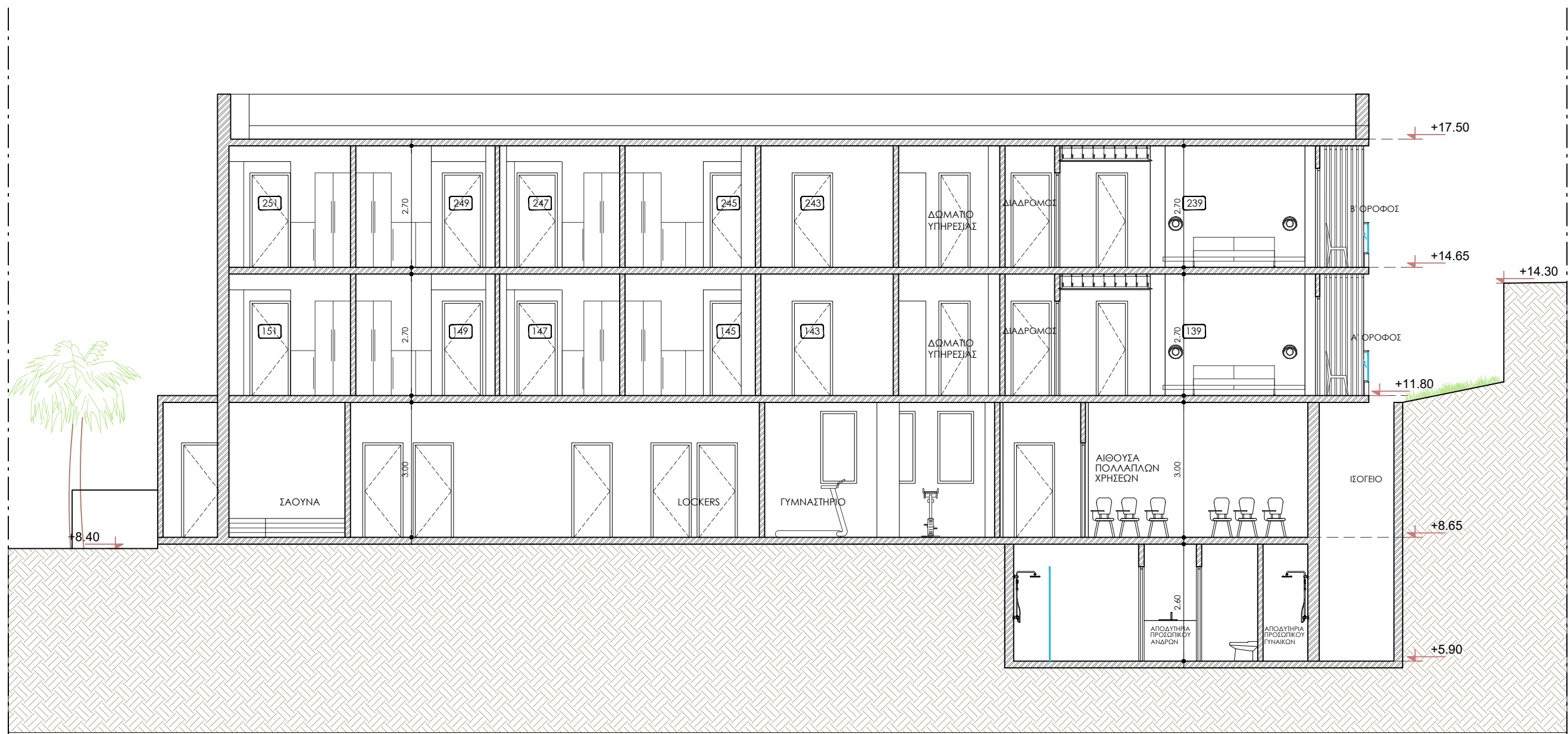
ΤΟΜΗ ΓΓ'
