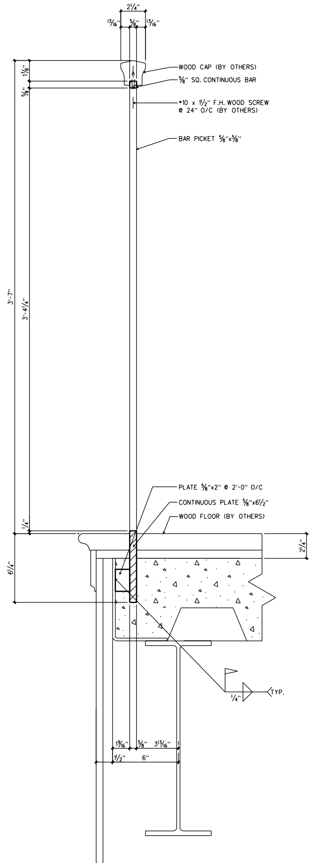
S1 SECTION SCALE: 3"=1'-0"
