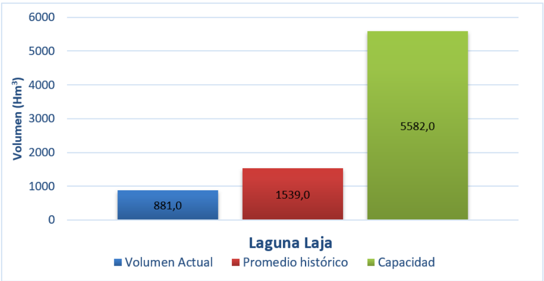
Figura 3.1. Volumen almacenado en Laguna Laja al 30 de junio 2026.
