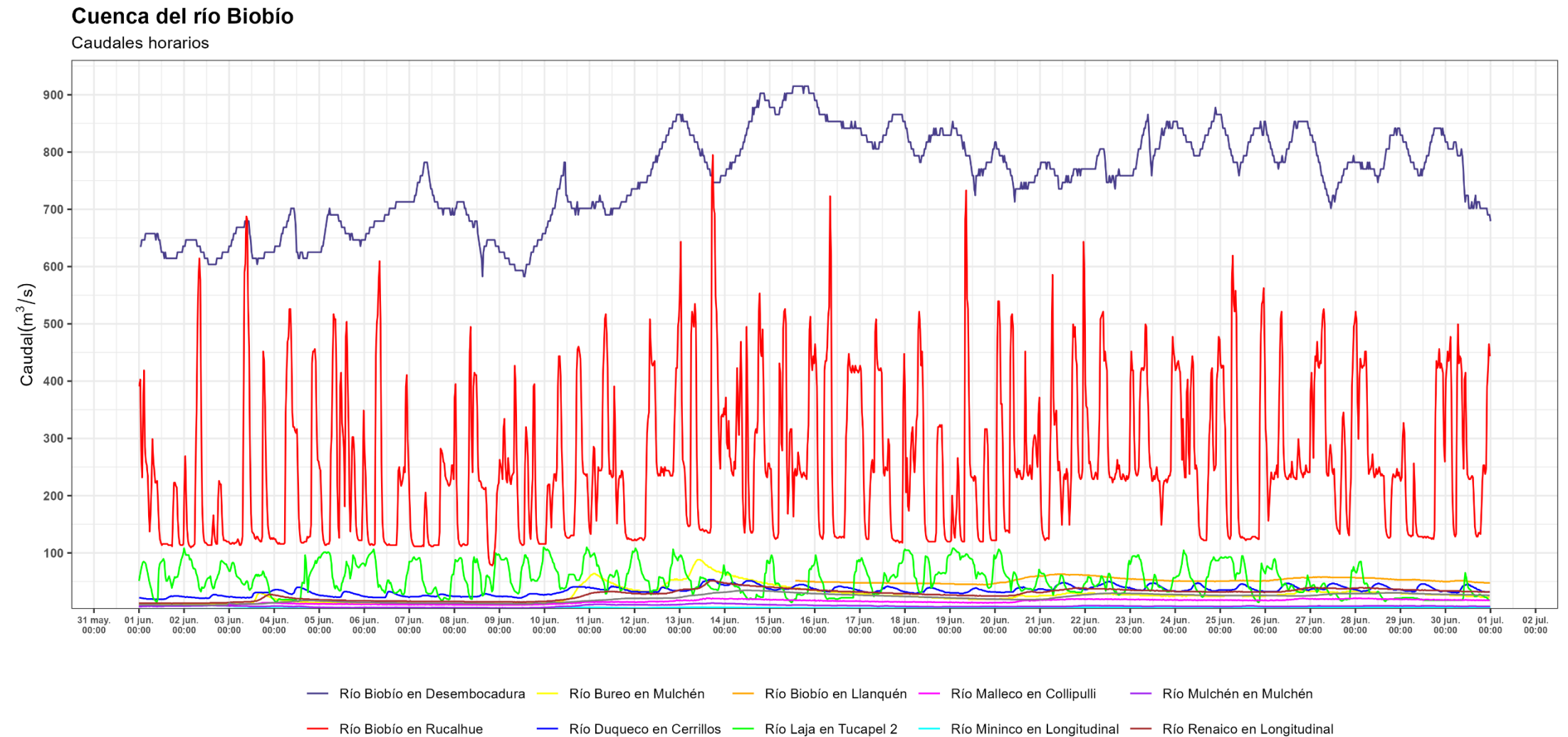
Figura 4.1. Hidrograma mes de junio 2026 en la cuenca del río Biobío
