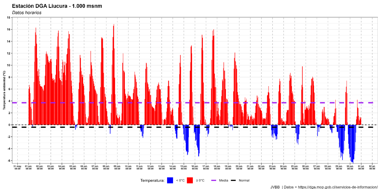
Figura 2.3.1. Variación de temperatura ambiental horaria junio 2026 DGA Liucura
