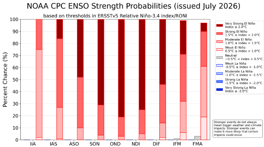
Figura 5.2.4: Pronóstico probabilístico ENSO para periodo junio 2026 – abril 2027.
