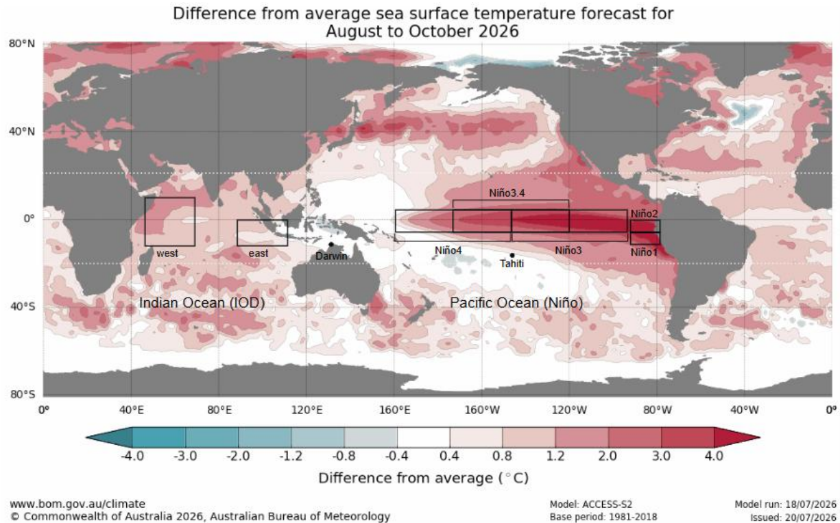
Figura 5.2.2: Regiones SST en el pacífico ecuatorial, agosto – septiembre - octubre 2026
