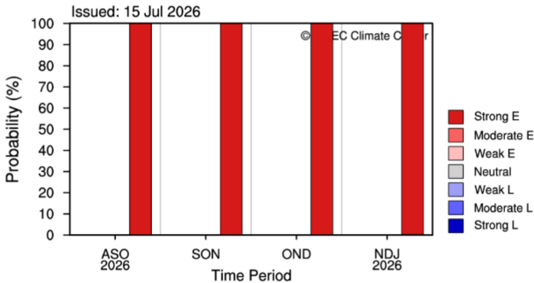
Figura 5.2.3: Pronóstico probabilístico ENSO para periodo agosto 2026 – enero 2027.
