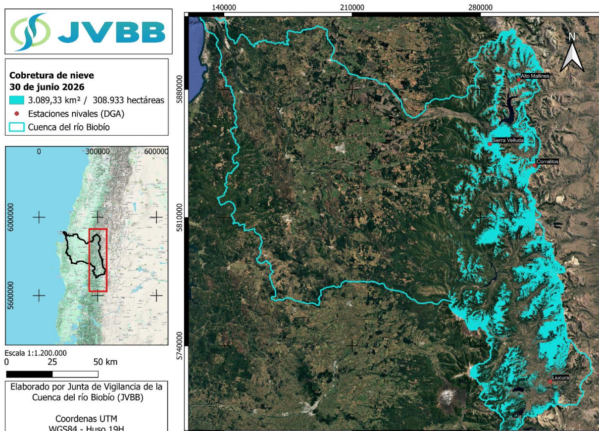
Figura 2.1.1. Cobertura nival en la cuenca del río Biobío al 30 de junio 2026.
