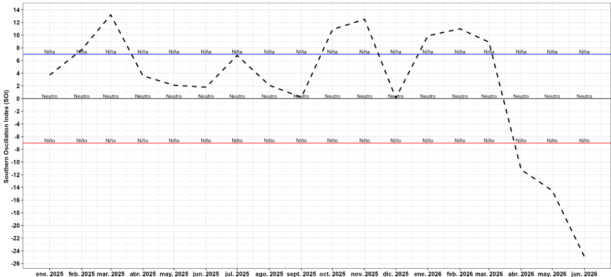
Figura 5.2.5: Índice de Oscilación del Sur al 30 de junio.
