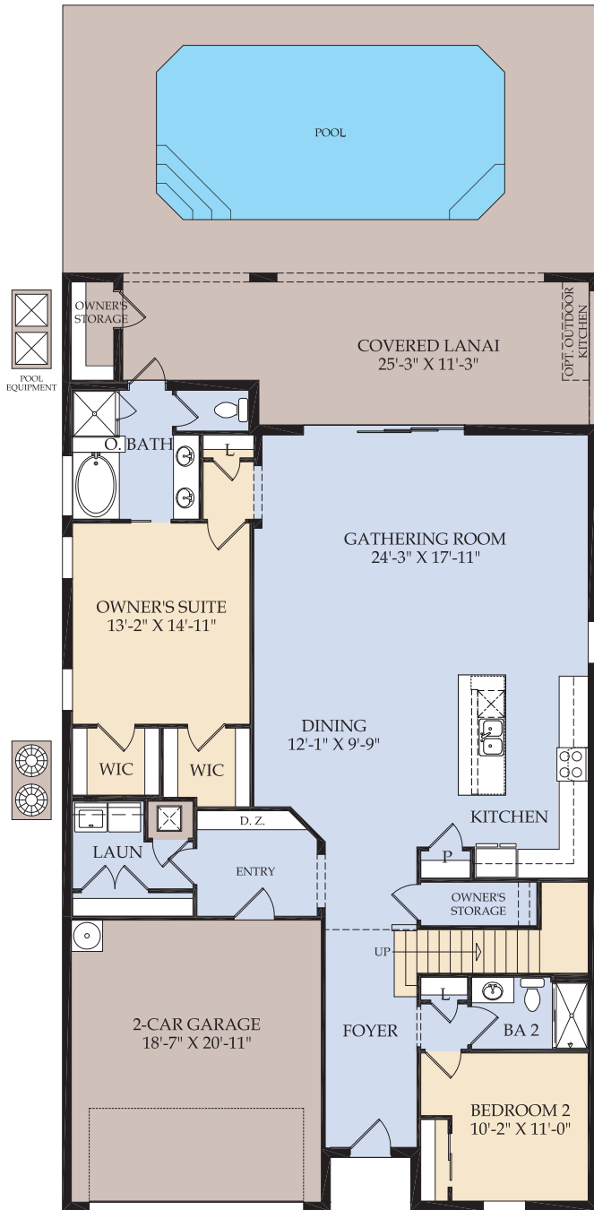
Primer piso
