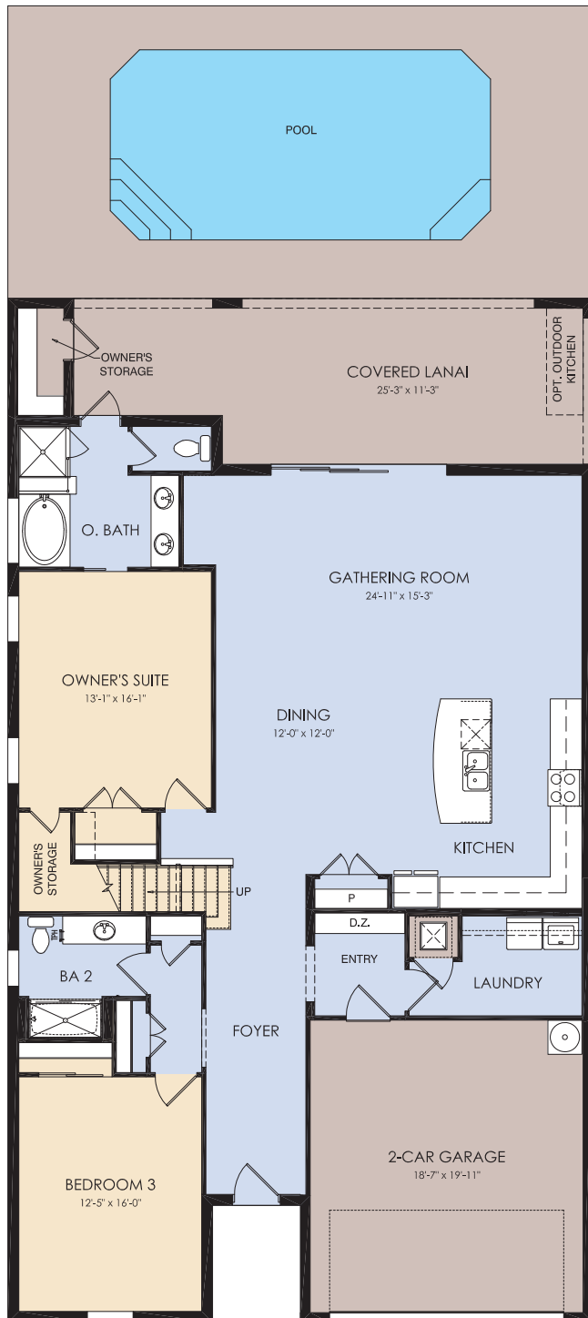
Primer piso
