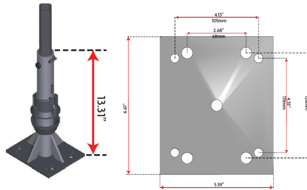
Base Cuplock para Ruedas
