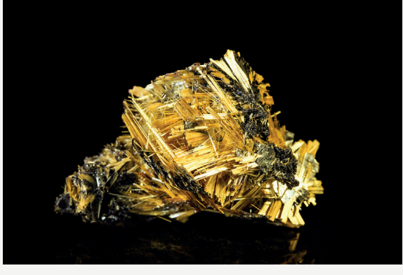
Rutile
