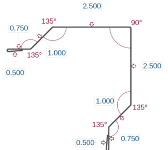
Mini Corner (MCRN)
