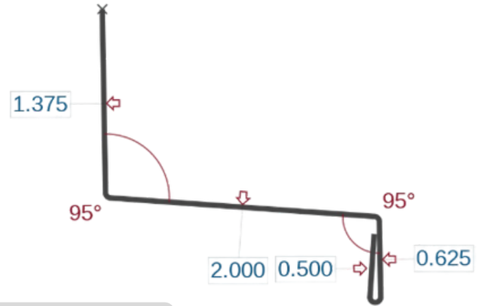
2" Double Angle (DA)
