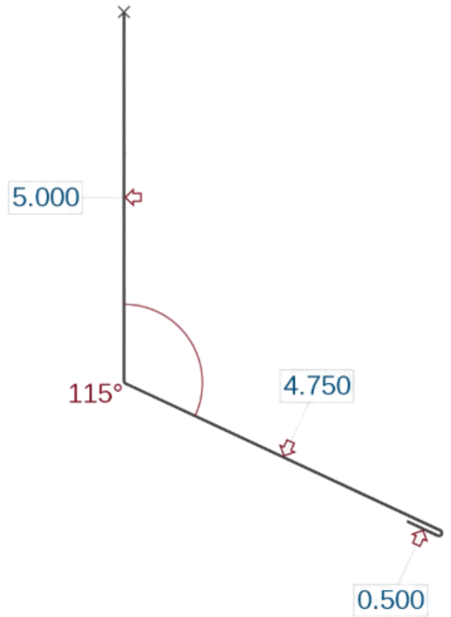
Universal Endwall (EWT)
