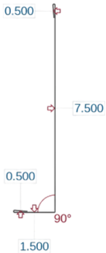
Fascia 7 1/2" (FT75)
