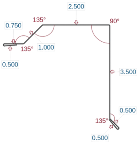
Mini Residential Rake Trim (RRTM)
