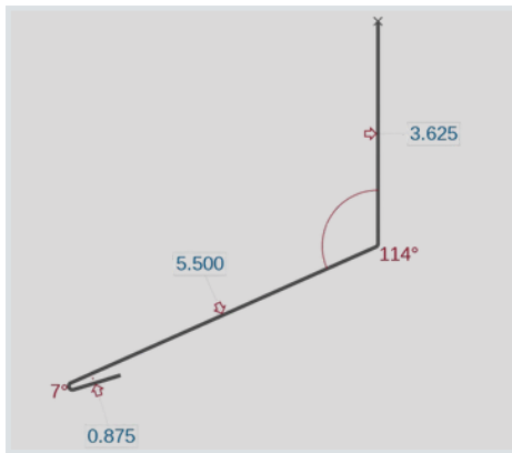
1.75 Z Clouser (ZC1)
