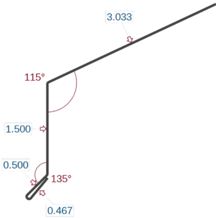
A Style Drip Edge
