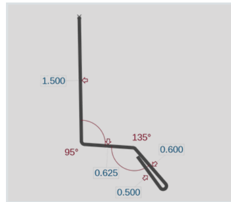
SB Top J (SBCTJ)
