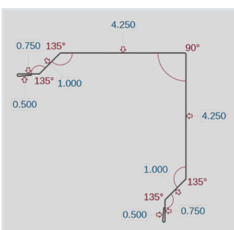
J-Channel (JT)
