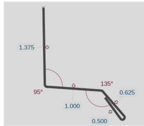
Top J (TJ)
