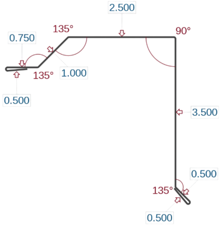
Mini Residential Rake Trim (RRTM)
