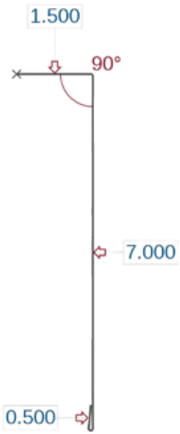
7" Door Post Trim (DJ7)
