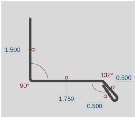
7.2 Top J (TJ72)
