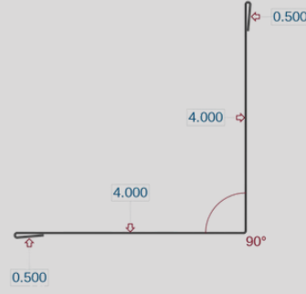
Soffit Top J (SFCTJ)
