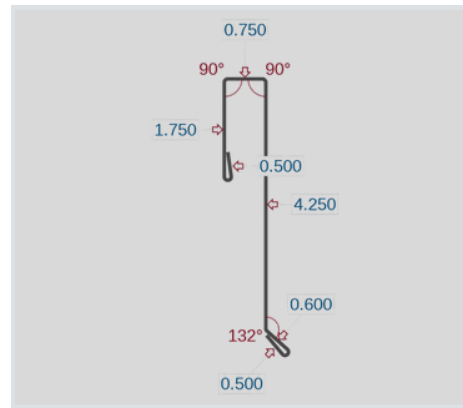
1.75 Sidewall (SW1)
