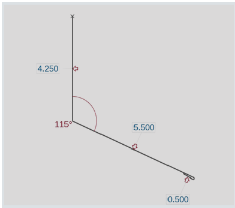
Snow Guard (SG)
