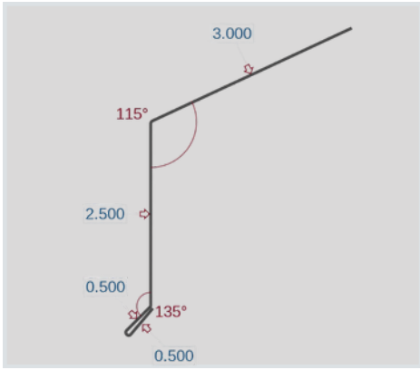
7.2 End Wall (EW72)
