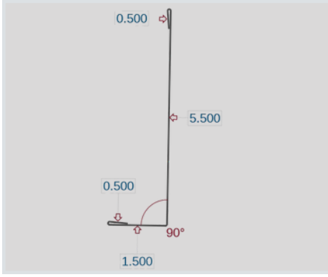
BB Fascia 5 1/2" (BBFT55)
