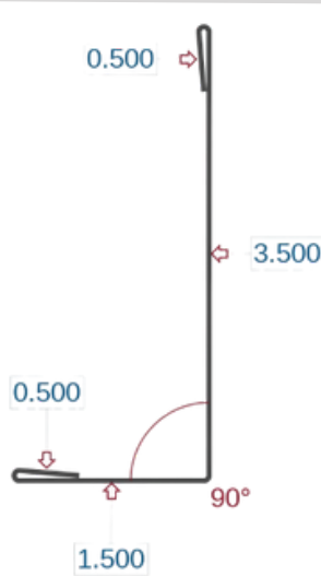
Fascia 3 1/2" (FT35)
