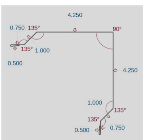
J-Channel (JT)
