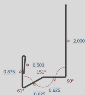
Soffit Top J (SFCTJ)
