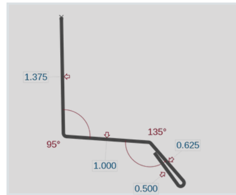
BB FJ Channel (BBFJ)
