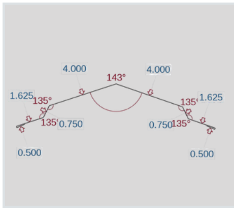
Universal Sidewall (SWT)
