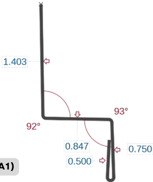
2" Double Angle (DA)
