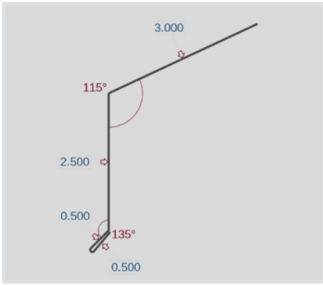
Universal Endwall (EWT)
