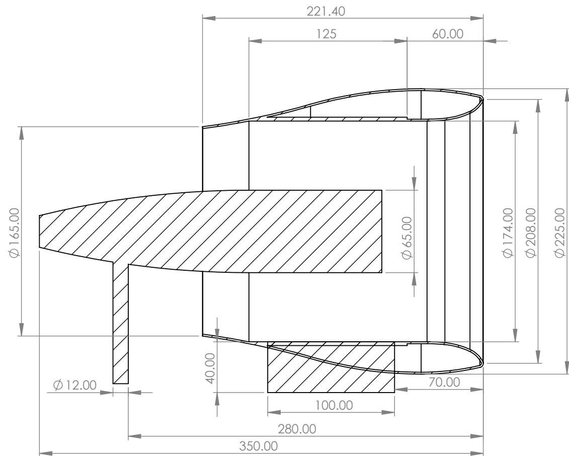
SECTION A-A SCALE 1 : 3
