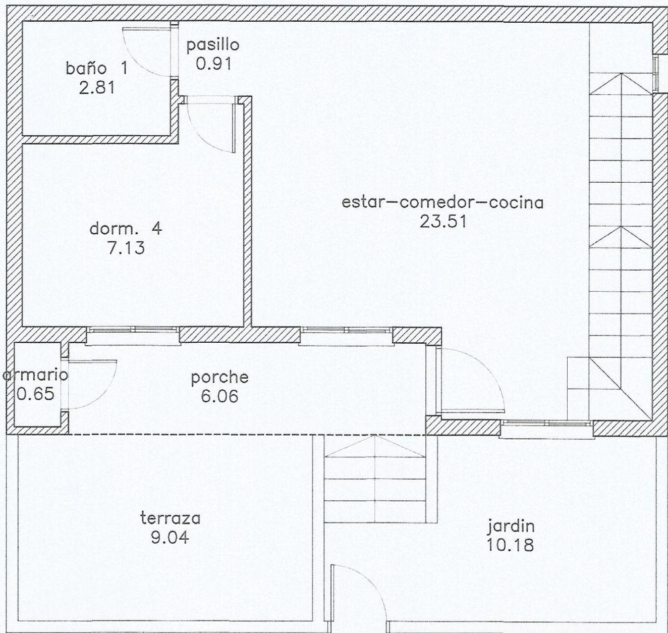
PLANTA BAJA
