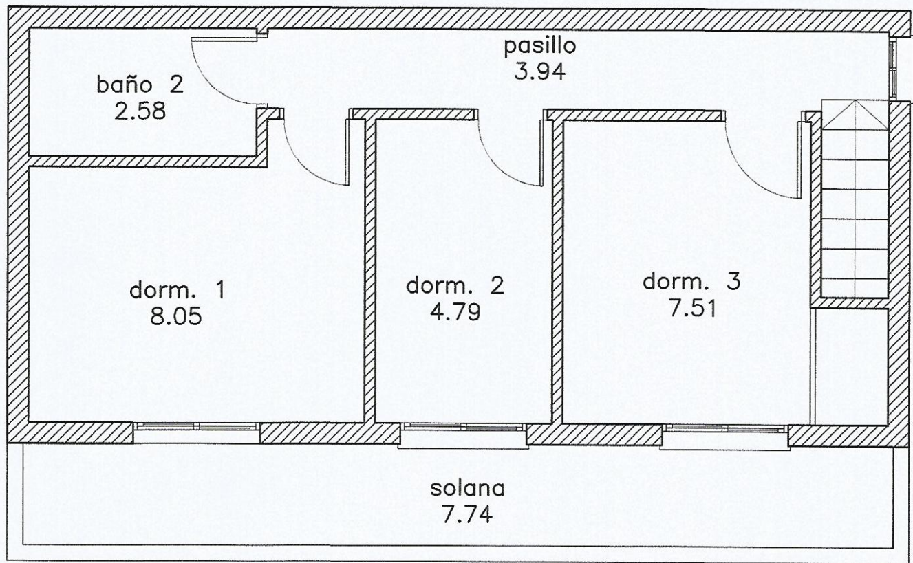
PLANTA PISO
