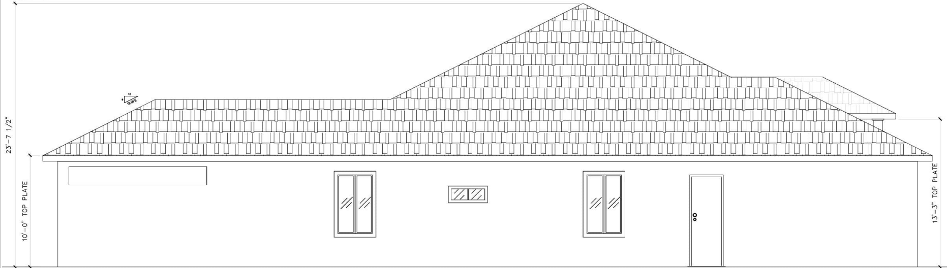
REAR ELEVATION SCALE: 3/8" = 1'-0"
