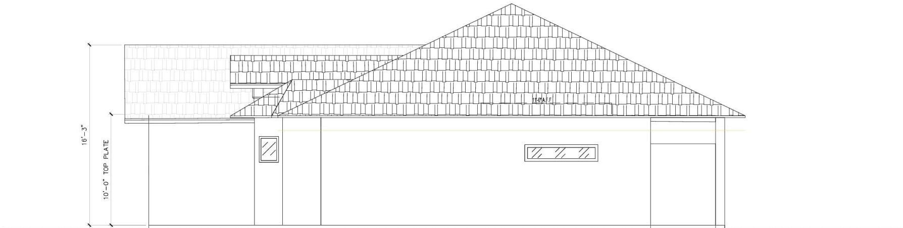
RIGHT ELEVATION SCALE: 3/8" = 1'-0"
