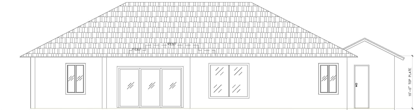
REAR ELEVATION SCALE: 3/8" = 1'-0"
