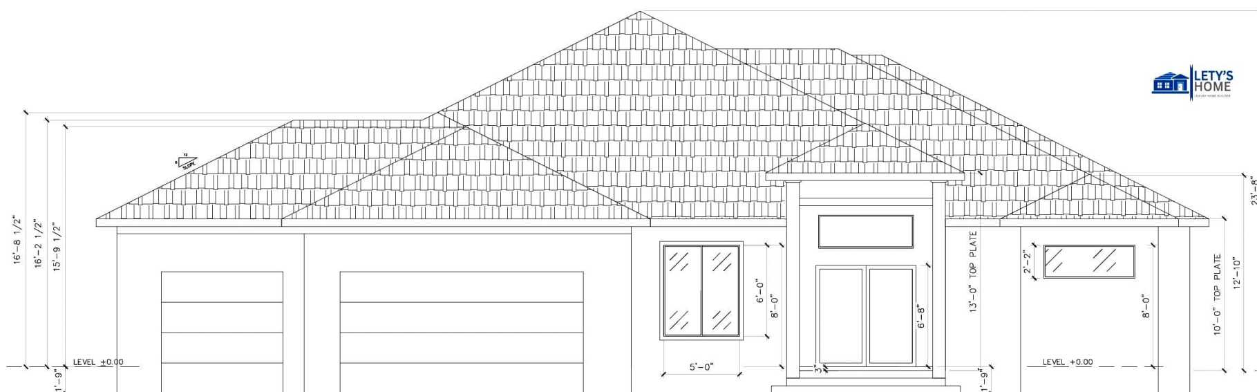
SCALE: 3/8" = 1'-0"
