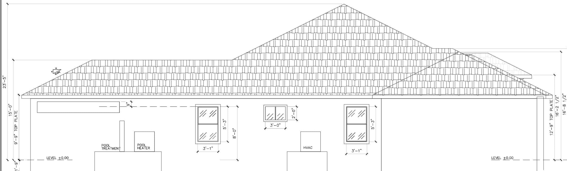
LEFT ELEVATION SCALE: 3/8" = 1'-0"
