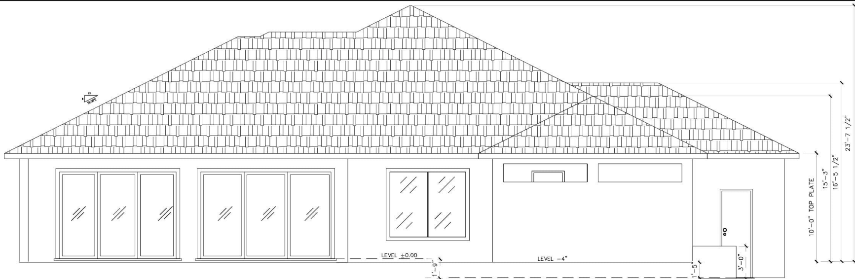
REAR ELEVATION SCALE: 3/8" = 1'-0"
