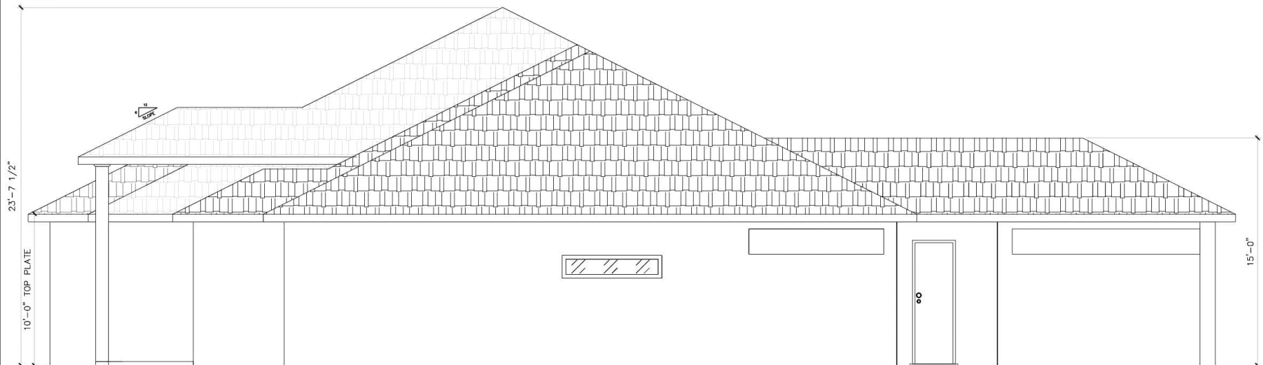
FRONT ELEVATION SCALE: 3/8" = 1'-0"
