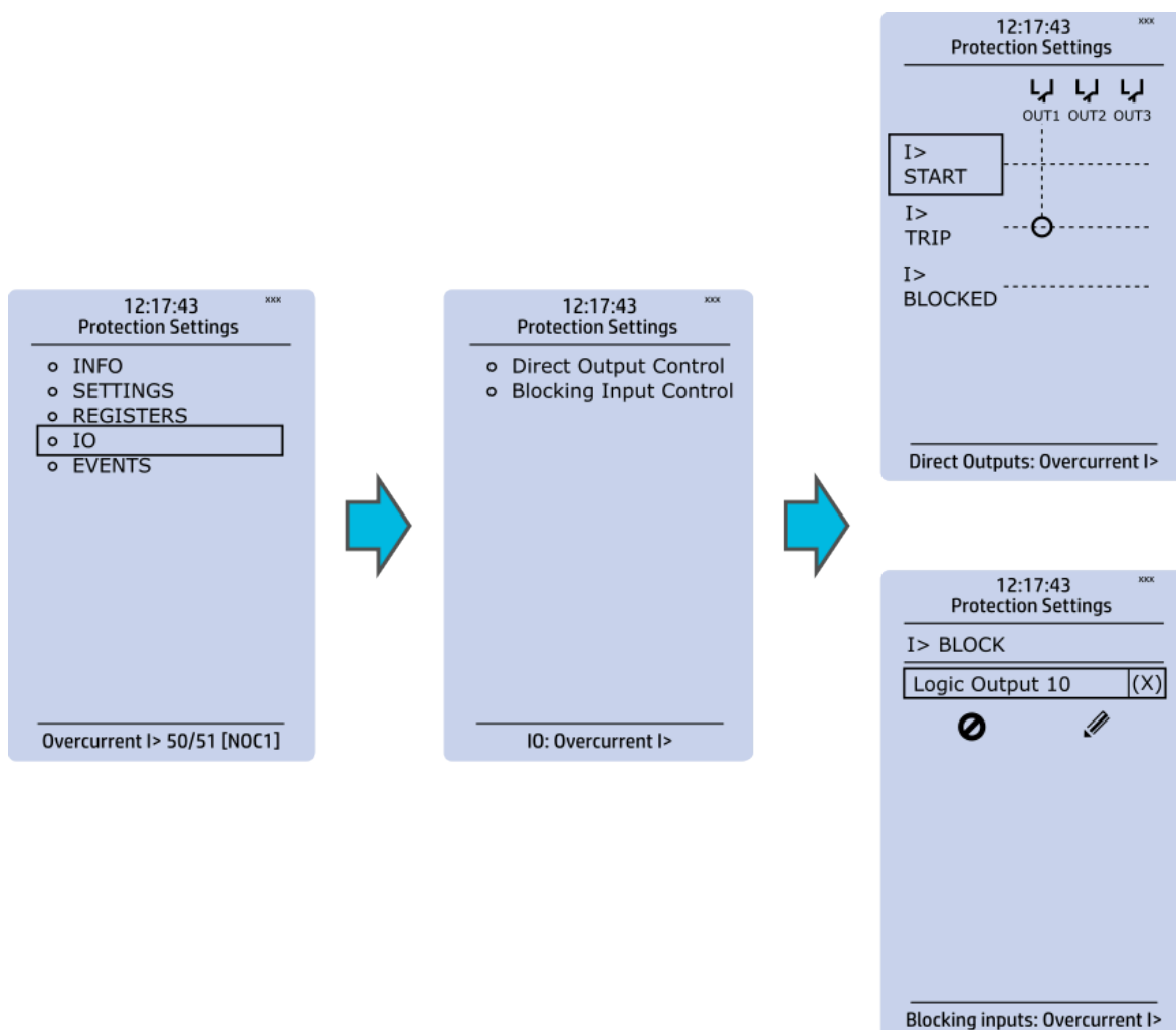
Figure. 3.4 - 14. I/O.
