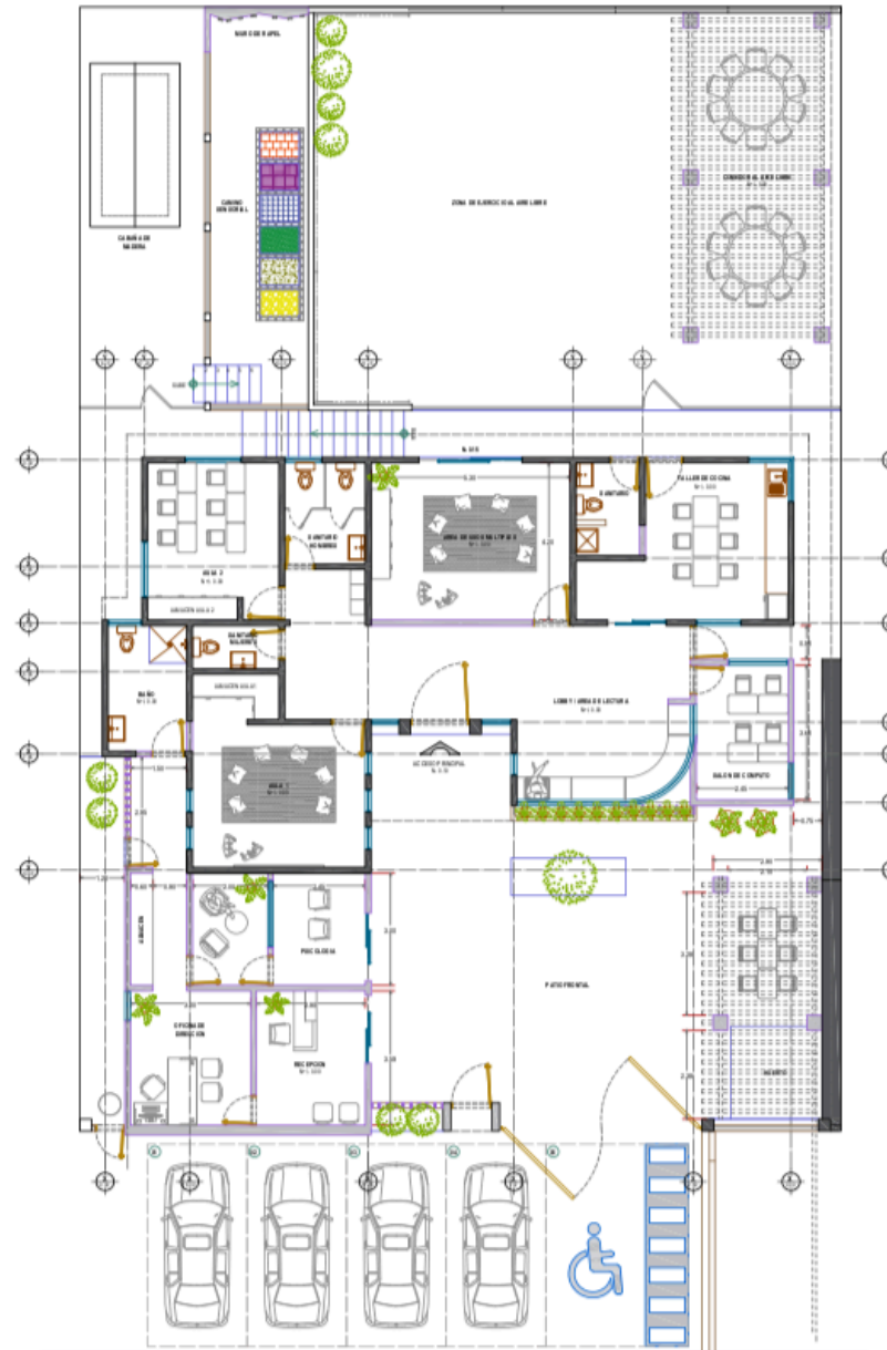
PLANTA ARQUITECTONICA ESC. 1:100
