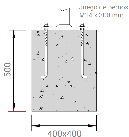
Vista - ALZADO
