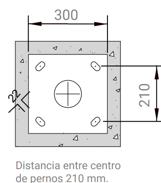
Vista - PLANTA
