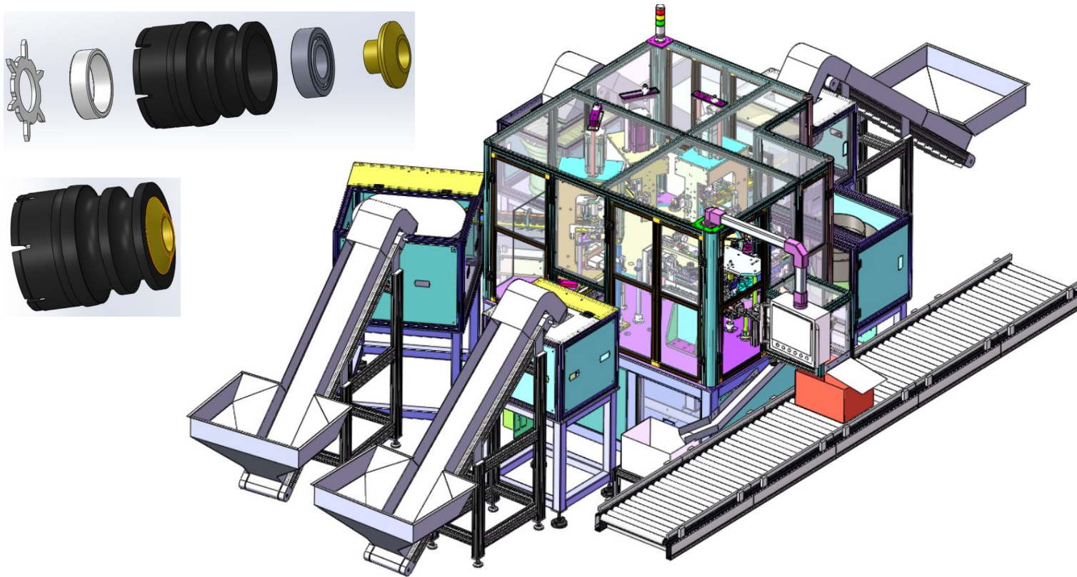
Línea de ensemble automática para tapa del roller 端盖自动组装线 Automatic assembly line for rollers' end cap
