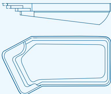
TIERRA 8 8.50 x 3.95 m | Prof. 0.90/1.70 m
