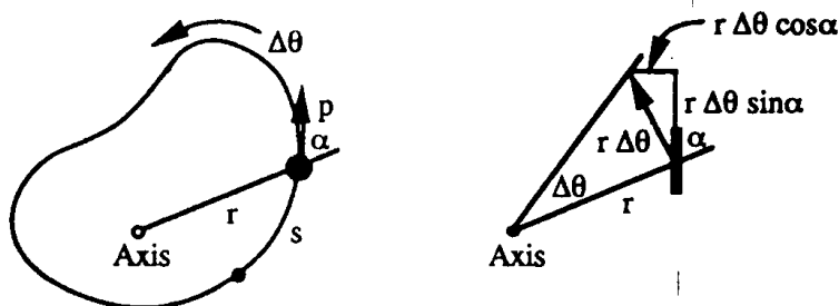
Fig. 9.07. Hannay hoop
