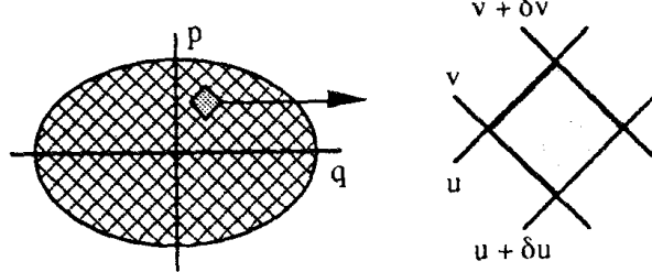
Fig. 7.03. Parametrizing the surface
