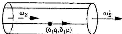
Fig. 10.02. Tube of trajectories
