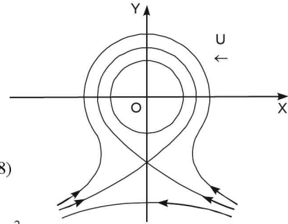
Fig. (iii) |k| > 4\pi aU
