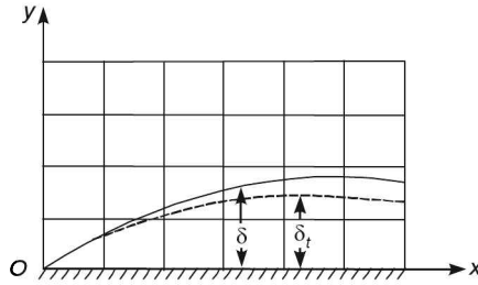
Fig. (iii) Pr > 1
