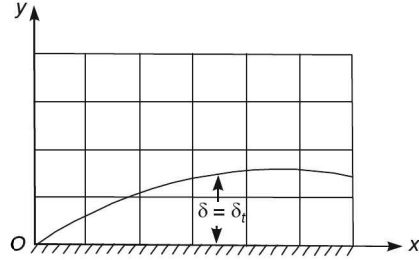
Fig. (ii) Pr = 1
