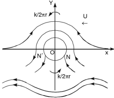
Fig. (i) |k| < 4\pi aU
