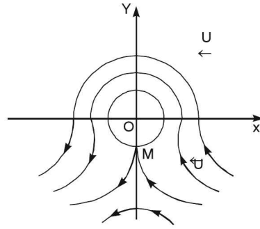
Fig. (ii) |k| = 4\pi aU
