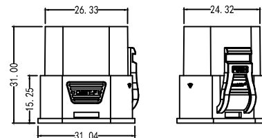
QS6T-F(公壳母端)
