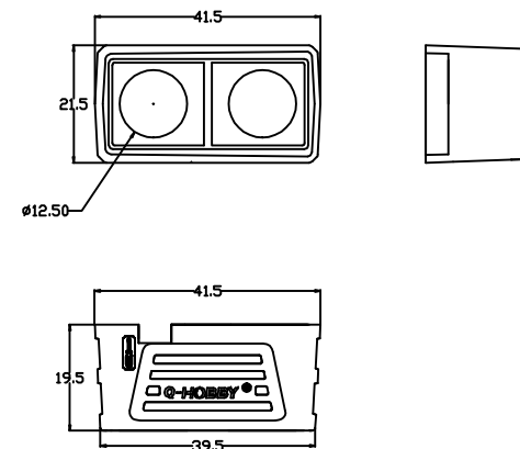
QS10P-L 护套
