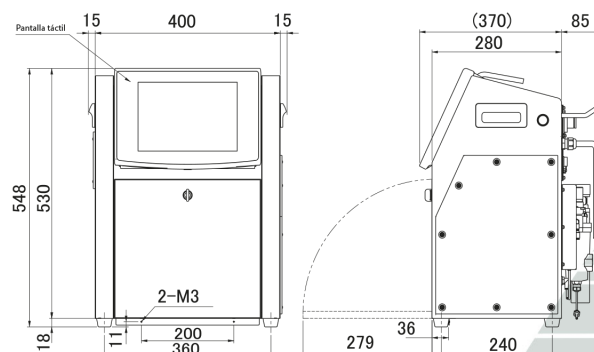
Cuerpo principal: 400 x 280 x 532mm.
