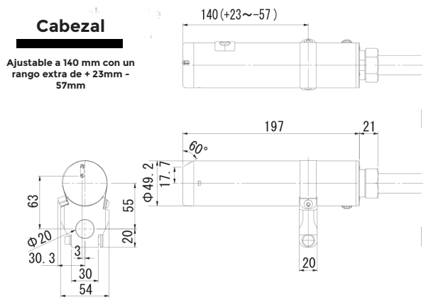
Cabezal de impresión: 49.2mm x 197mm.
