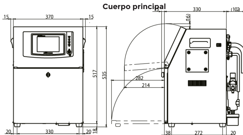
Cuerpo principal: 400 x 280 x 532mm.
