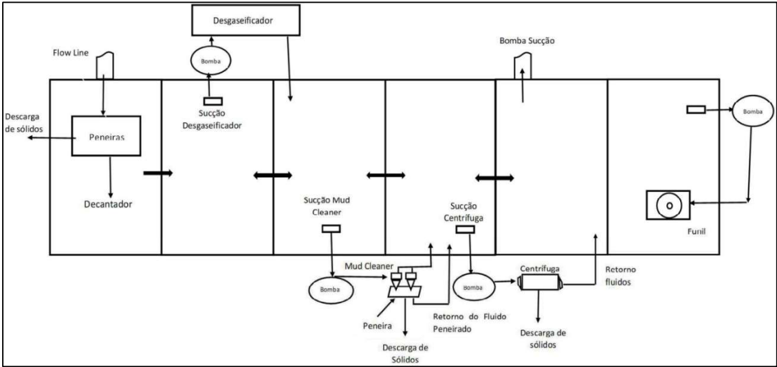
Figura 1 – Layout e arranjo proposto para os tanques da sonda e para o sistema extratores de sólidos
