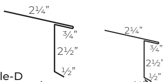
Style-D Style-D W/Hem
