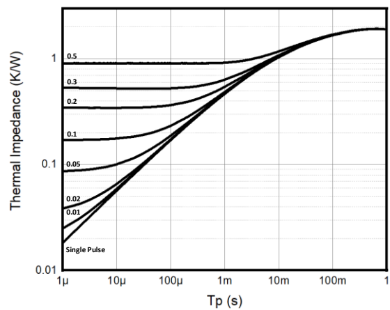
Fig. 8 Thermal Impedance
