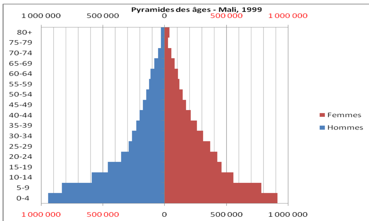
Figure 2 : pyramide des âges_Mali 1998
