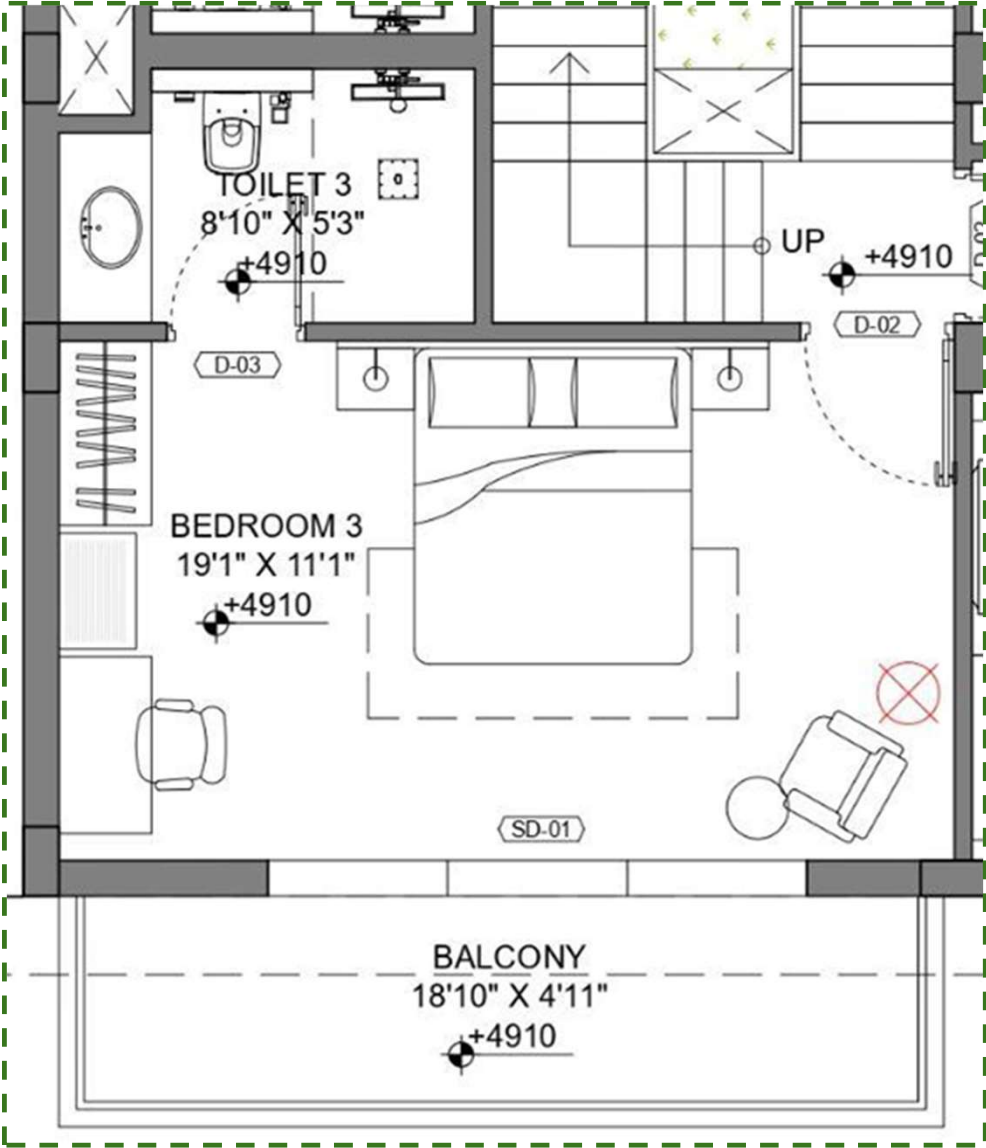
BEDROOM 3 - FF
