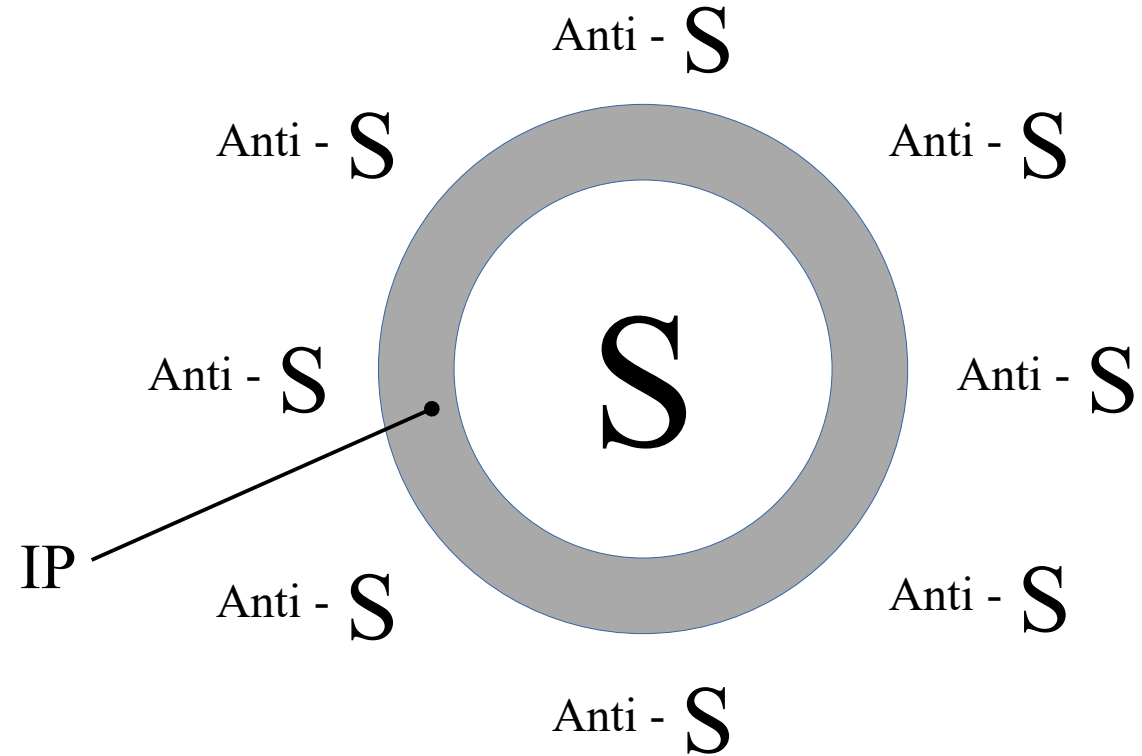
Limites do espaço amostral para insights S + \sim S = 1
