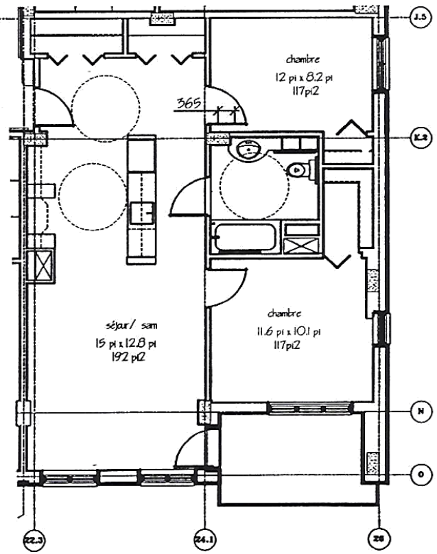
Plan de logement type 2 inversé
