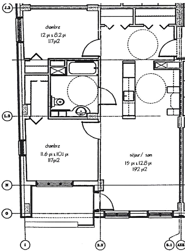
Plan de logement type 2
