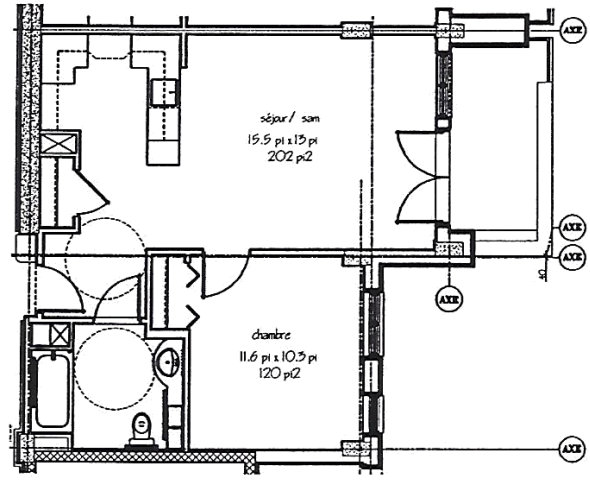
Plan du logement type 3
