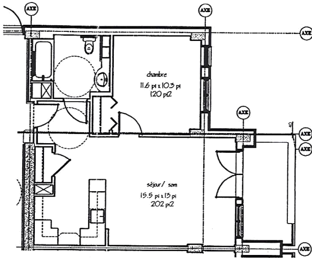
Plan du logement type 3 inversé
