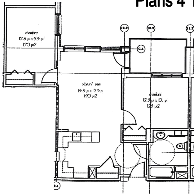
Plan du logement type 4
