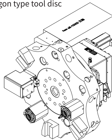
多邊形刀盤 Polygon type tool disc
