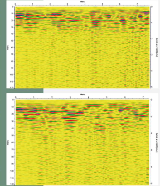
P43 (5.00 m) ve P44 (5.00 m) nolu profil ölçümleri ve düşey radargram kesitleri.
